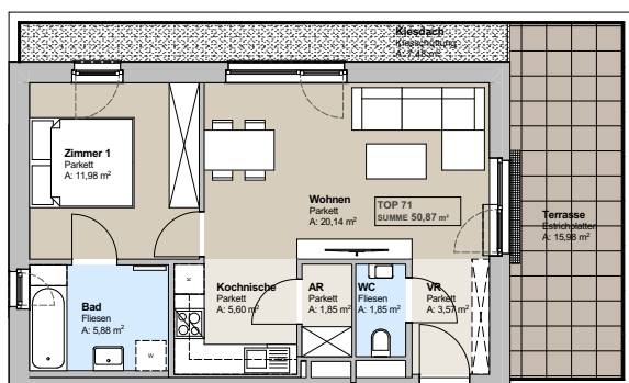
Grundrissbeispiel
