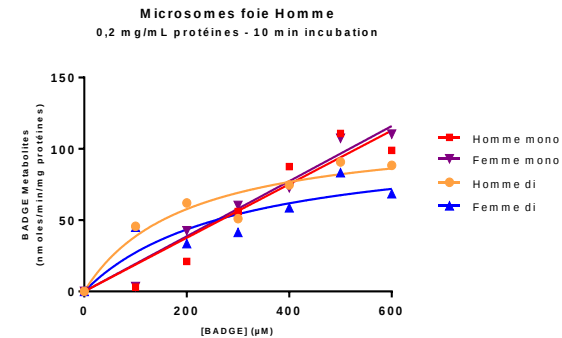
Fig. 7 et 8. A gauche, radio-HPLC d'une incubation de [14C]-BADGE (100 \mu\text{M} , 4h) avec des micro-tranches de foie de rat : formation du BADGE mono-H 2 O et du BADGE di-H 2 O; A droite, formation de ces métabolites lors d'incubations réalisées avec des fractions microsomales hépatiques humaines.
