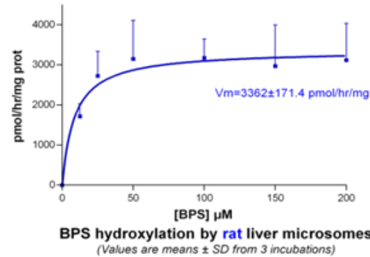
Figure 6. Cinétique de formation du métabolite hydroxylé du BPS en fonction de la concentration de [3H]-BPS incubée avec des fractions microsomales hépatiques de rat (gauche) ou d'homme (centre)
