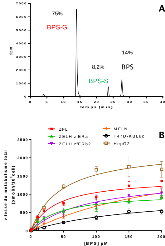
Figure 5 : A) Radio-chromatogramme caractéristique du métabolisme du BPS sur lignées cellulaires humaines (ici : HepaRG, 24h, 150 \mu\text{M} BPS) montrant les deux métabolites majoritaires : le BPS glucuronide (BPS-G) et le BPS sulfate (BPS-S). B) Cinétique de métabolisation (globale : tous métabolites confondus) du BPS sur lignées cellulaires : HepG2, modèle hépatique, est une lignée métaboliquement compétente (Le Fol et al. 2016).
