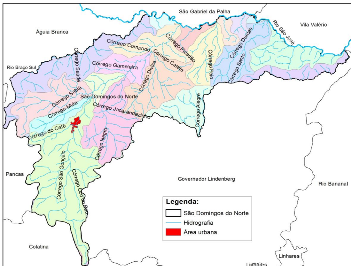
Figura 3-29 - Sub-bacias do município de São Domingos do Norte.
