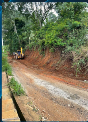
RECUPERAÇÃO DE ESTRADA Córrego Frio, Campo do Coelho
