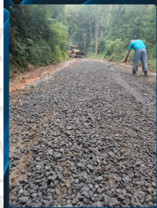
RECUPERAÇÃO DE ESTRADA Galdinópolis, Lúmiar
