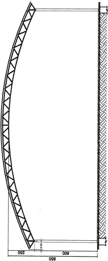
CORTE A-A Escala 1/125
