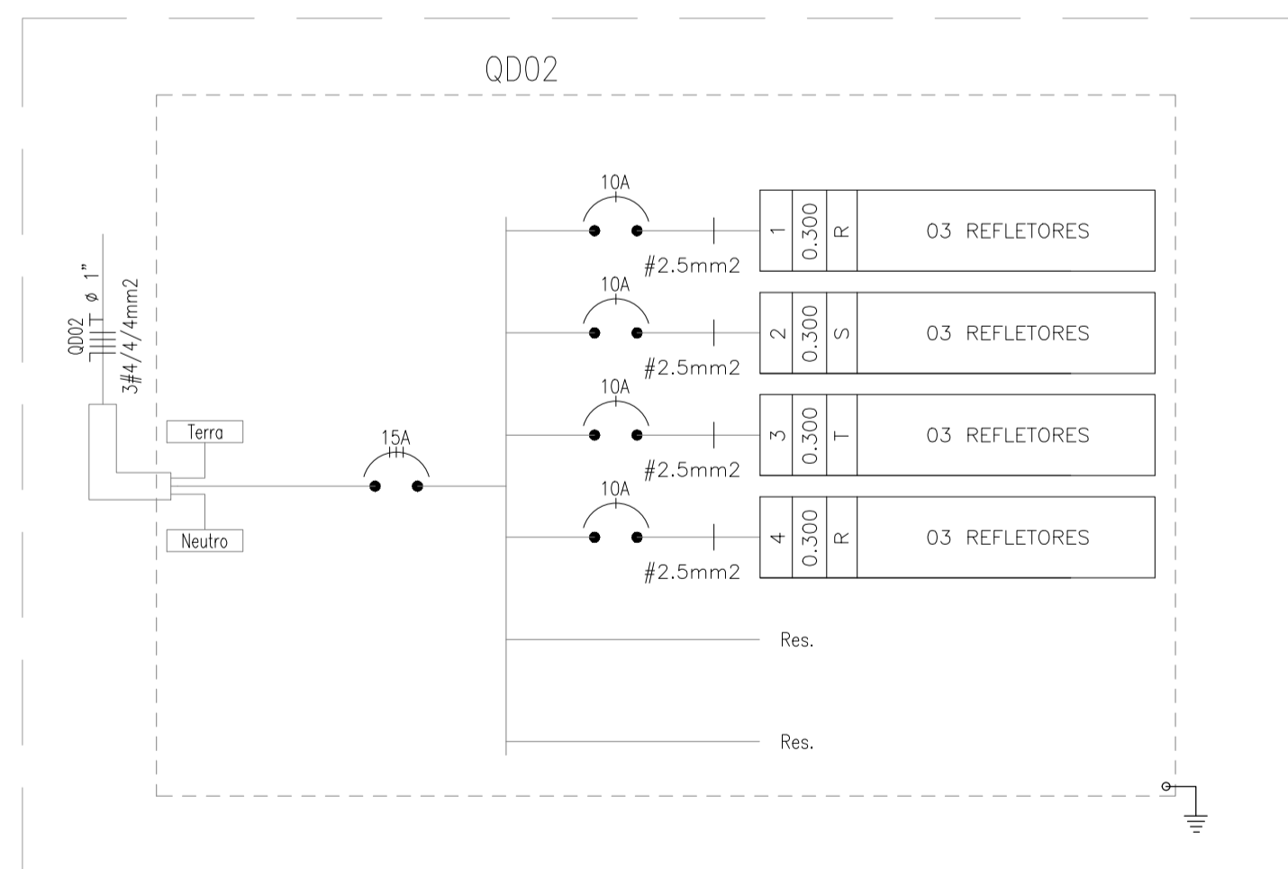
DIAGRAMA UNIFILAR ESC.:1/50
