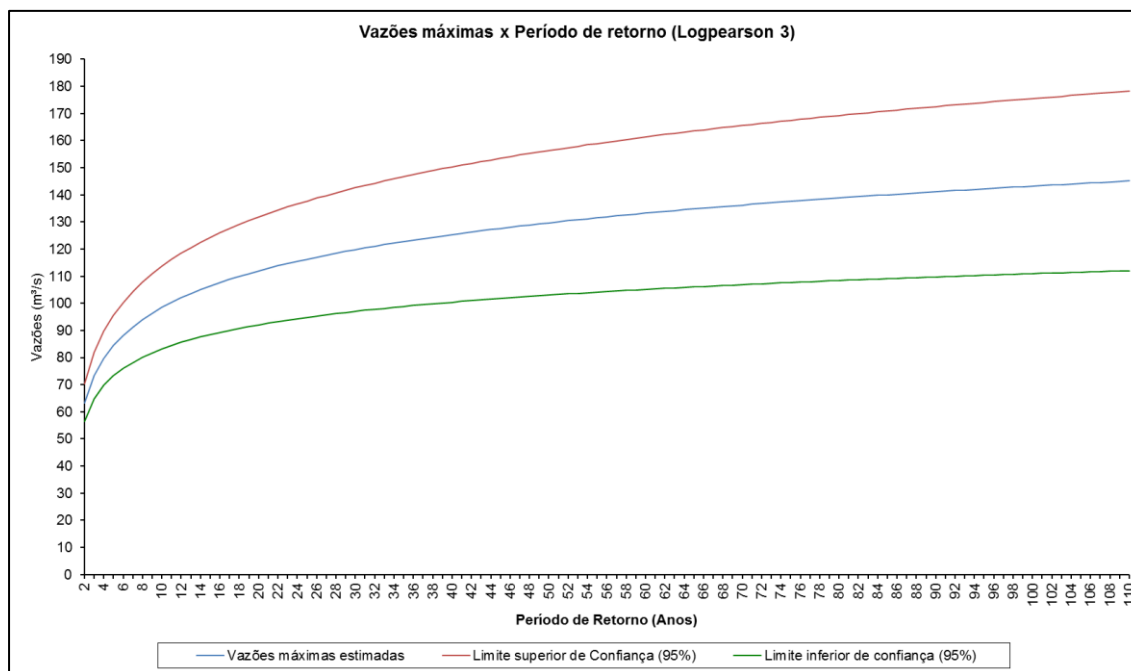
Figura 3-31 - Gráfico da vazão máxima associada a cada período de retorno estimada pela distribuição Logpearson 3 para a estação Córrego do Galo.
