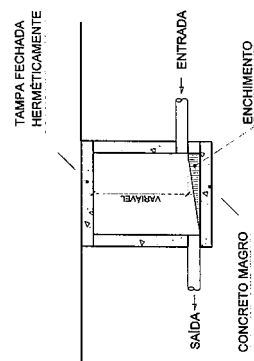
CORTE DA CX. DE INSPEÇÃO
