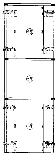
Armação negativa das lajes do pavimento Cobertura (Eixo Y)
