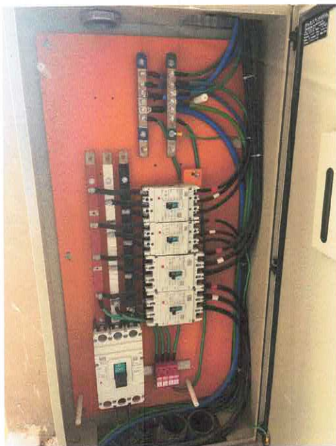
QUADRO -QGBT/DIJUNTORES/DPS/DR
