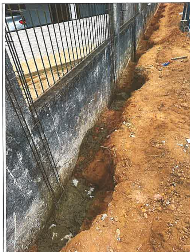
Foto 19 - Fornecimento e Colocação de Armadura e Fornecimento e Aplicação de Concreto
