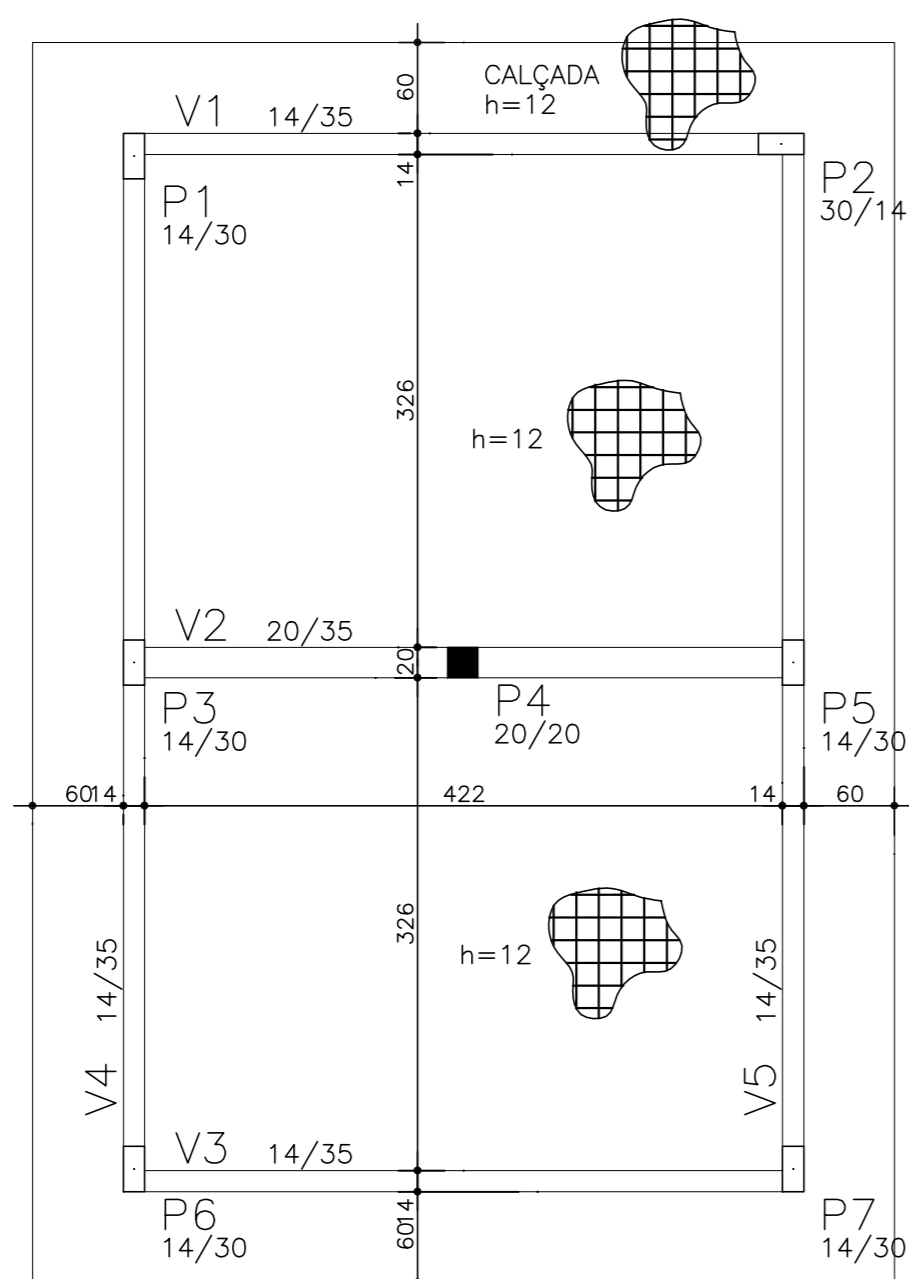
FORMA DO TERREO ESCALA 1/50
