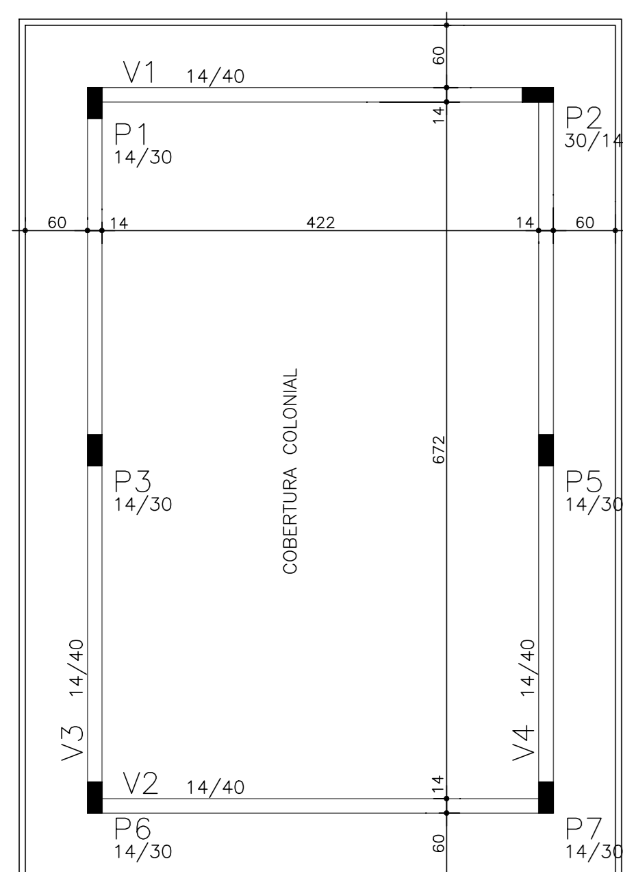
FORMA DA COBERTURA ESCALA 1/50
