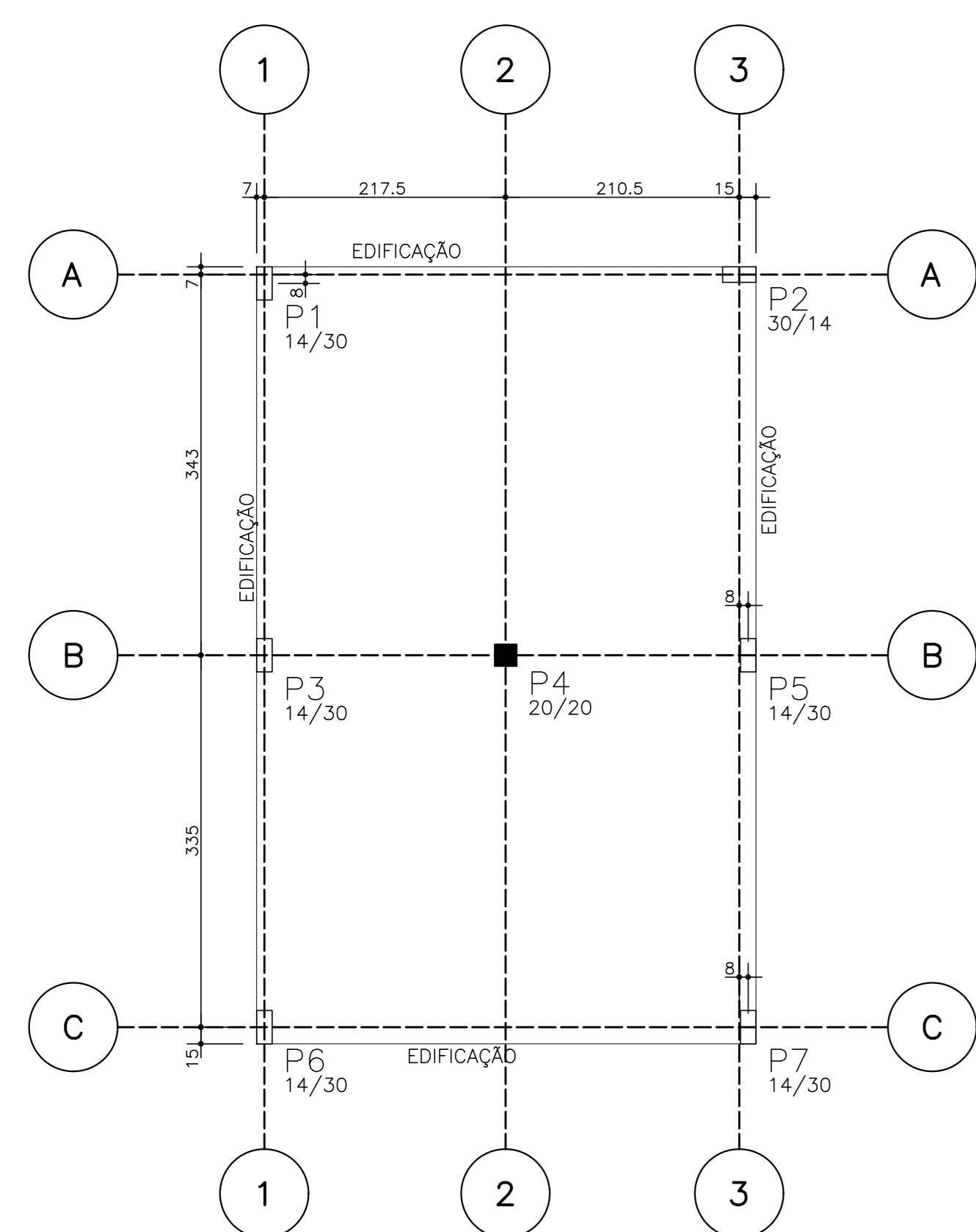
LOCAÇÃO DOS PILARES ESCALA 1/50
