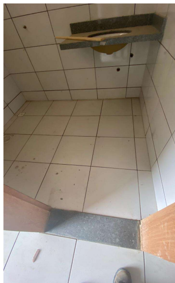
PISO CERÂMICO ANTIDERRAPANTE PEI V - 40 X 40 CM, E SOLEIRA EM GRANITO, LARGURA 15 CM, ESPESSURA 2,0 CM, ÁREA VEST. FUNCIONÁRIO
