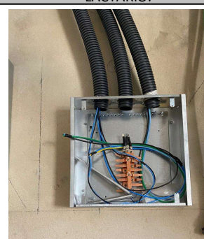
QUADRO DE DISTRIBUIÇÃO DE ENERGIA, DE EMBUTIR, COM 18 DIVISÕES MODULARES, COM BARRAMENTO - QD1
