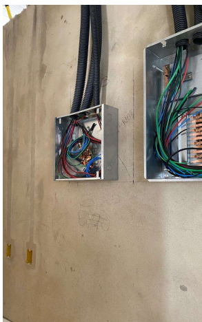
QUADRO DE DISTRIBUIÇÃO DE ENERGIA, DE EMBUTIR, COM 12 DIVISÕES MODULARES COM BARRAMENTO - QD3
