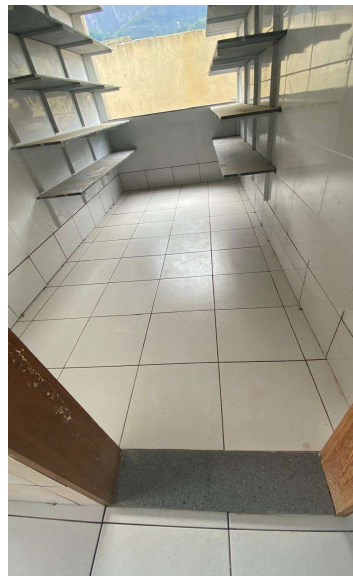
PISO CERÂMICO ANTIDERRAPANTE PEI V - 40 X 40 CM, E SOLEIRA EM GRANITO, LARGURA 15 CM, ESPESSURA 2,0 CM, ÁREA DESPENSA.
