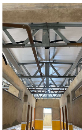
ELETROCALHA LISA TIPO U 150X75MM, E ELETROCALHA LISA COM TAMPA 100 X 50 MM - ÁREA DO BLOCO B
