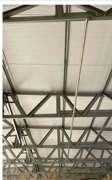
ELETRODUTO DE AÇO GALVANIZADO, CLASSE LEVE, DN 25 MM (1), APARENTE, INSTALADO EM TETO - ÁREA DO PÁTIO COBERTO.
