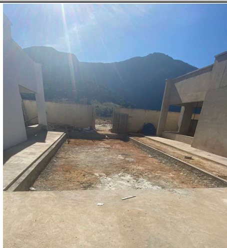
CAIXA DE AREIA EM ALVENARIA DE VEDAÇÃO DE BLOCOS CERÂMICOS MACIÇOS DE 5X10X20CM (ESPESSURA 10CM) E ARGAMASSA DE ASSENTAMENTO COM PREPARO EM BETONEIRA.
