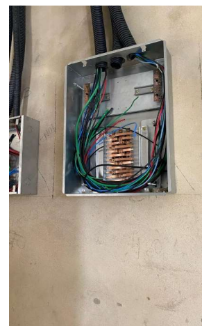
QUADRO DE DISTRIBUIÇÃO DE ENERGIA, DE EMBUTIR, COM 24 DIVISÕES MODULARES, COM BARRAMENTO - QD2
