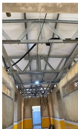
ELETROCALHA LISA TIPO U 150X75MM, E ELETROCALHA LISA COM TAMPA 100 X 50 MM - ÁREA DO BLOCO B
