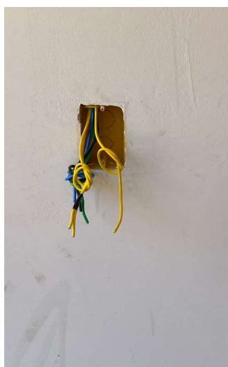
CABO DE COBRE FLEXIVEL ISOLADO, ANTI-CHAMA 450/750 V, PARA CIRCUITOS TERMINAIS
