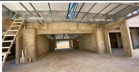
FOTO 14 - TELHA SANDUICHE METALICA COM PREENCHIMENTO EM PIR 30MM, 0,5 X 0,43 MM.
