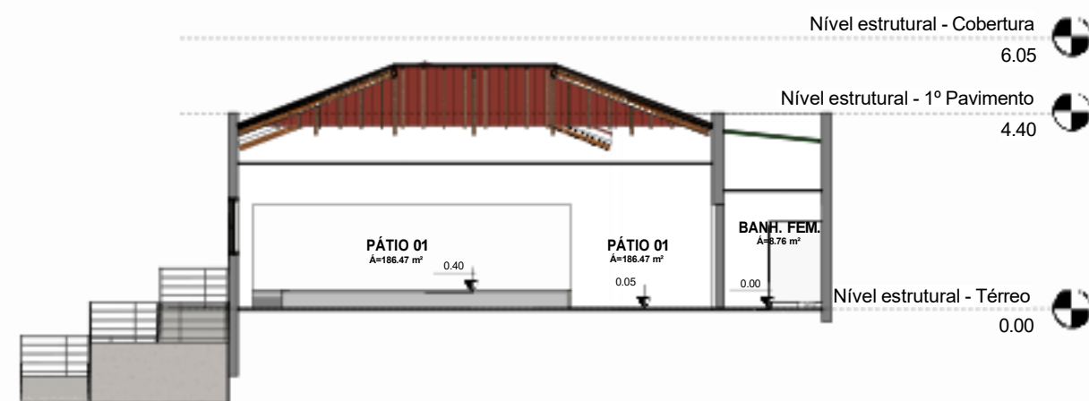
4 CORTE C - C 1 : 100
