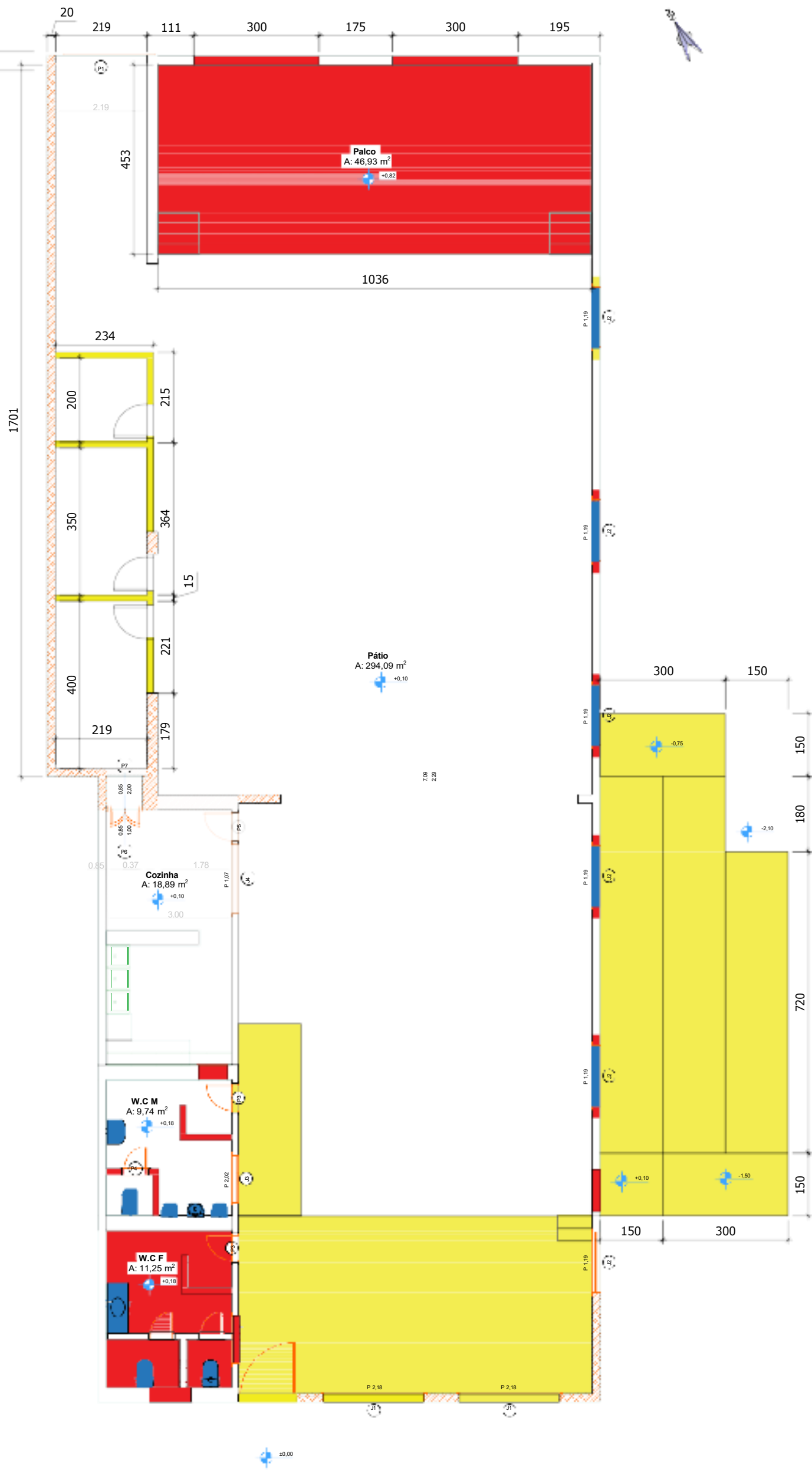
PLANTA FAIXA - DEMOLIÇÕES, RETIRADAS E CONSTRUÇÃO
