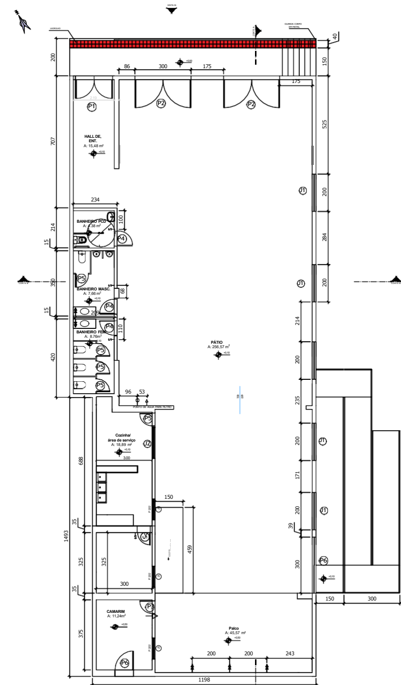
PLANTA BAIXA E INDICAÇÕES DE PONTOS ELÉTRICOS ESC.: 1/100
