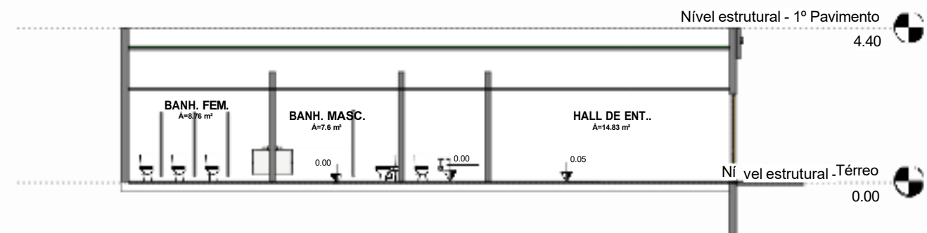
3 CORTE B - B 1 : 100
