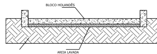
DETALHE ESQUEMATICO - PAVIMENTAÇÃO DE VIAS ESC: 5/ESCALA
