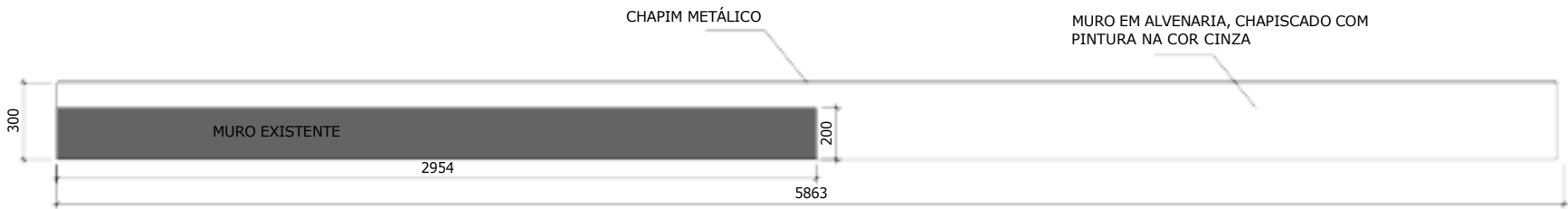
CONSTRUÇÃO DE MURO (FACHADA FACHADA LATERAL ESQUERDA). ESC: 1/125
