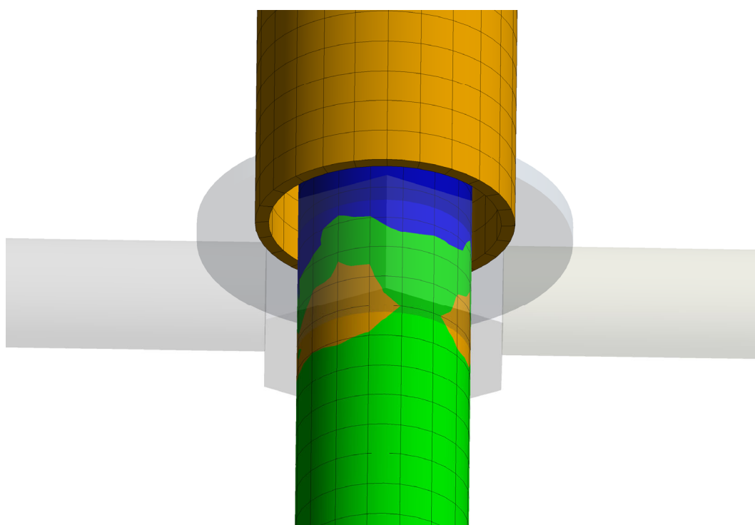
Figura 5 – Fator de segurança para o carregamento LC1 na estrutura.
