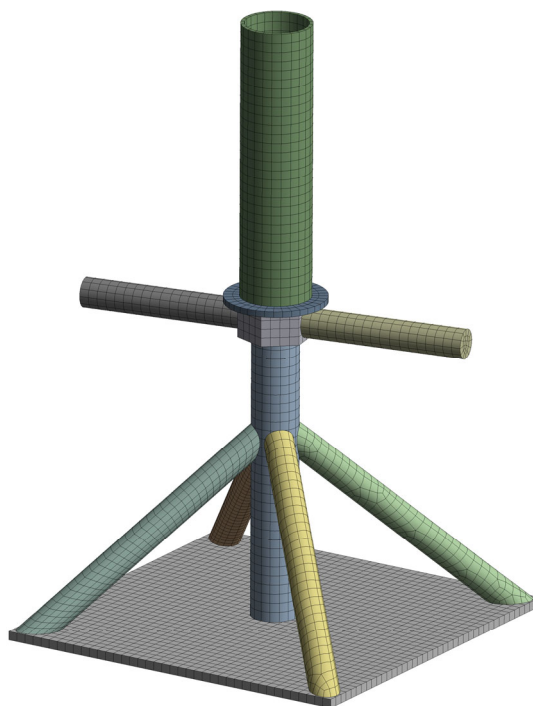
Figura 3 – Malha gerada para o modelo em estudo.
