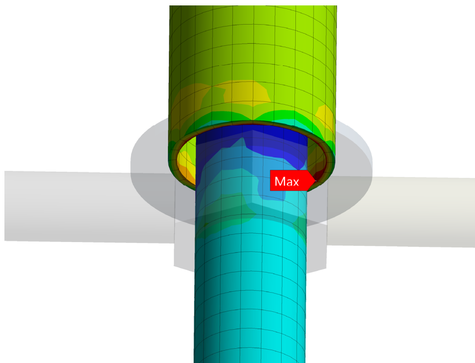
Figura 7 - Tensão de von-Mises calculada em MPa para o carregamento LC1 na estrutura.
