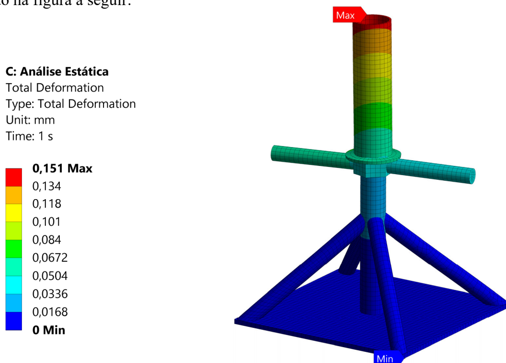
Figura 4 - Deslocamento estrutural o carregamento LC1 na estrutura calculado em mm.
