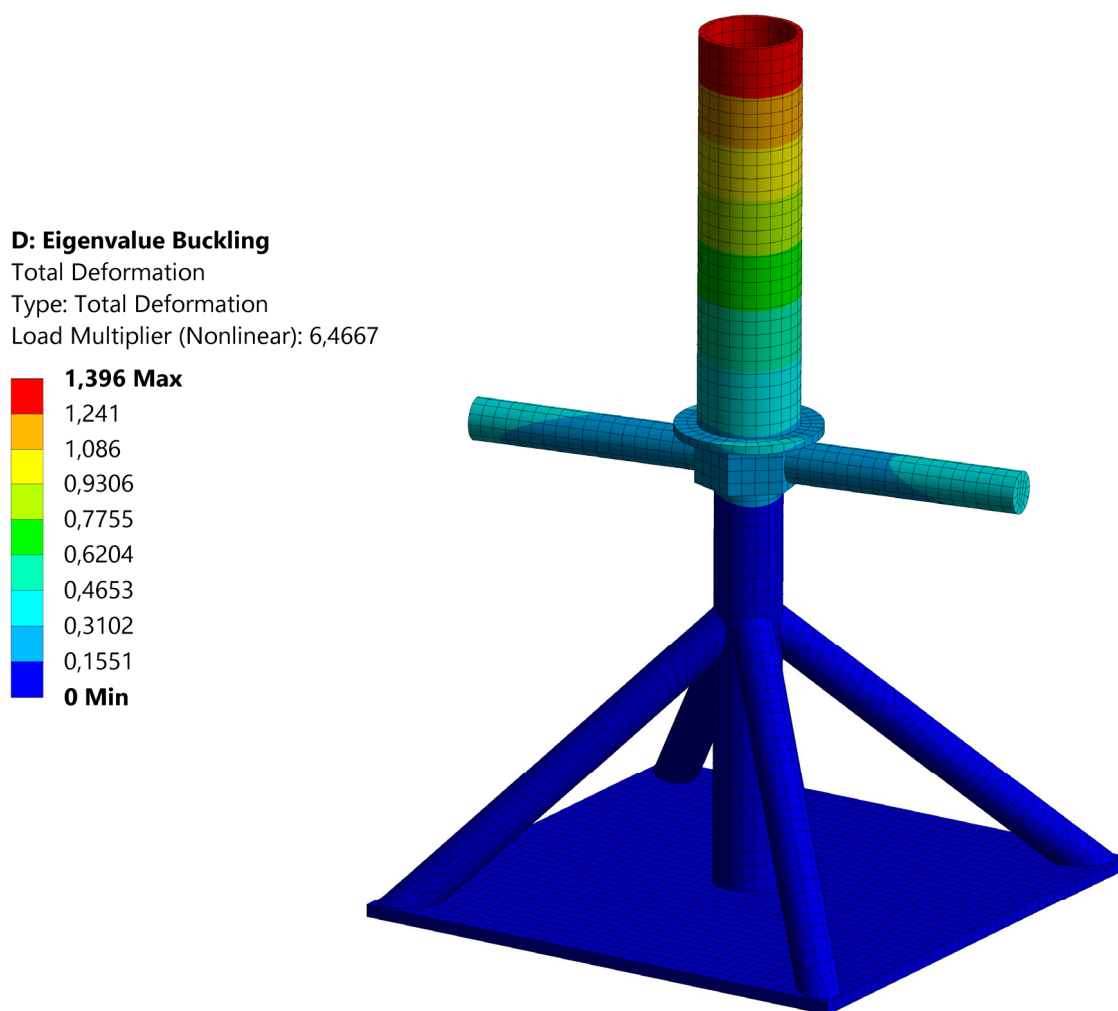
Figura 6 – Primeiro modo de flambagem para o carregamento LC1 na estrutura.
