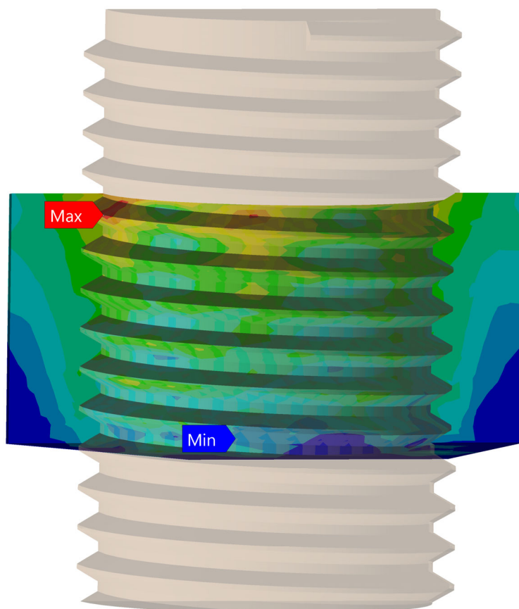
Figura 8 - Tensão de von-Mises calculada em MPa para o contato entre barra roscada e porca.
