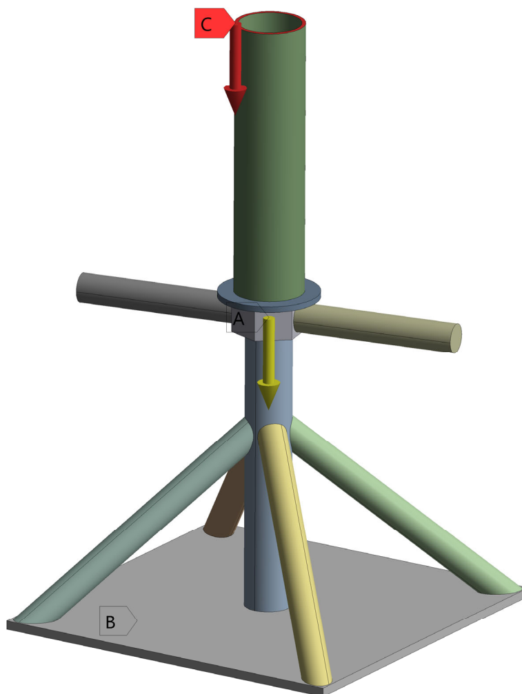
Figura 2 – Cargas e condições de contorno para o carregamento LC1.
