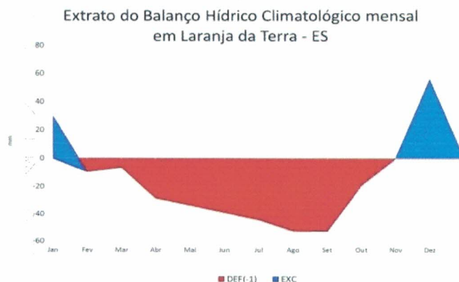
Figura 6: Extrato do balanço hídrico climatológico. Fonte: Elaborados pela Coordenação de Meteorologia.
