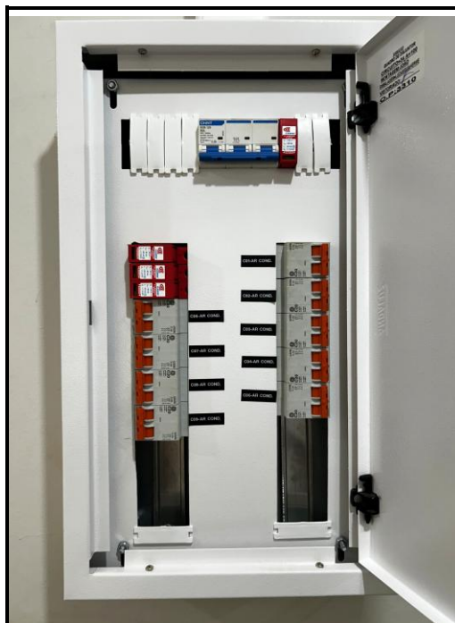
Foto 02: QD1 - Quadro Ar Condicionado
