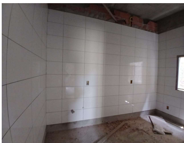
Foto 11: Execução de revestimento de parede
