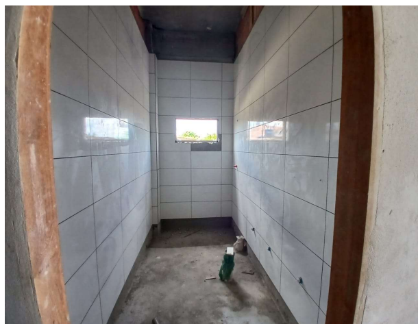
Foto 19: Execução de revestimento de parede
