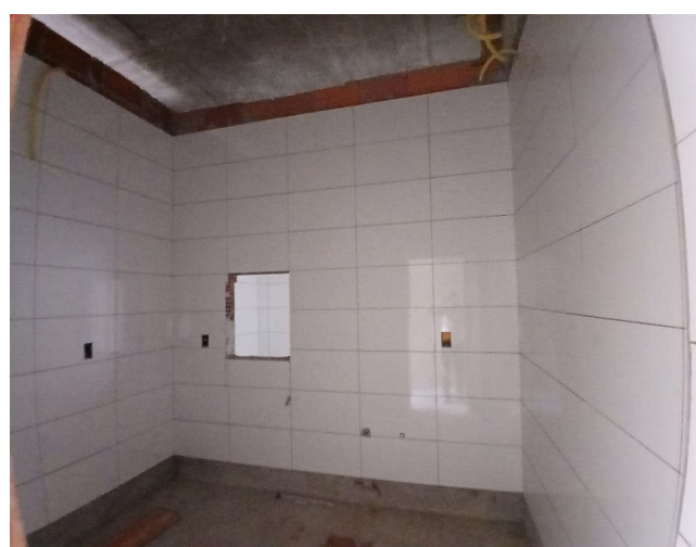
Foto 16: Execução de revestimento de parede
