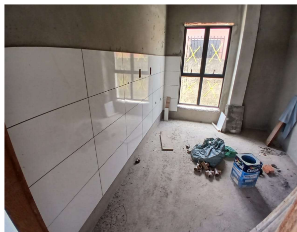
Foto 18: Execução de revestimento de parede
