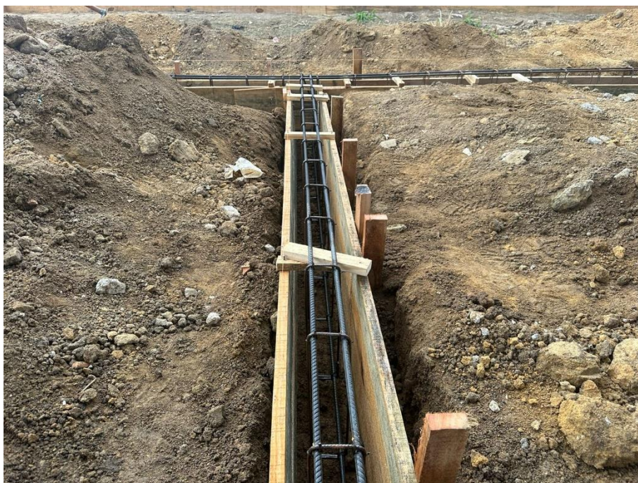
Foto 14 – Cintas do vestiário com fôrmas e suas devidas ferragens (ITENS 20.04, 20.05 e 20.06)
