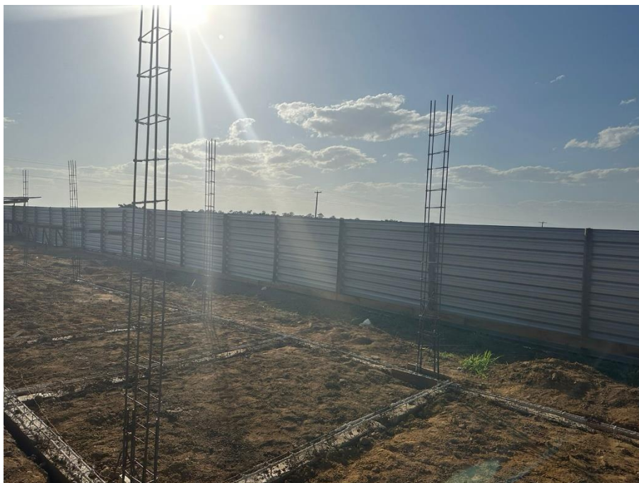
Foto 15 – Ferragem dos pilares do vestiário instalados (ITENS 20.05 e 20.06)
