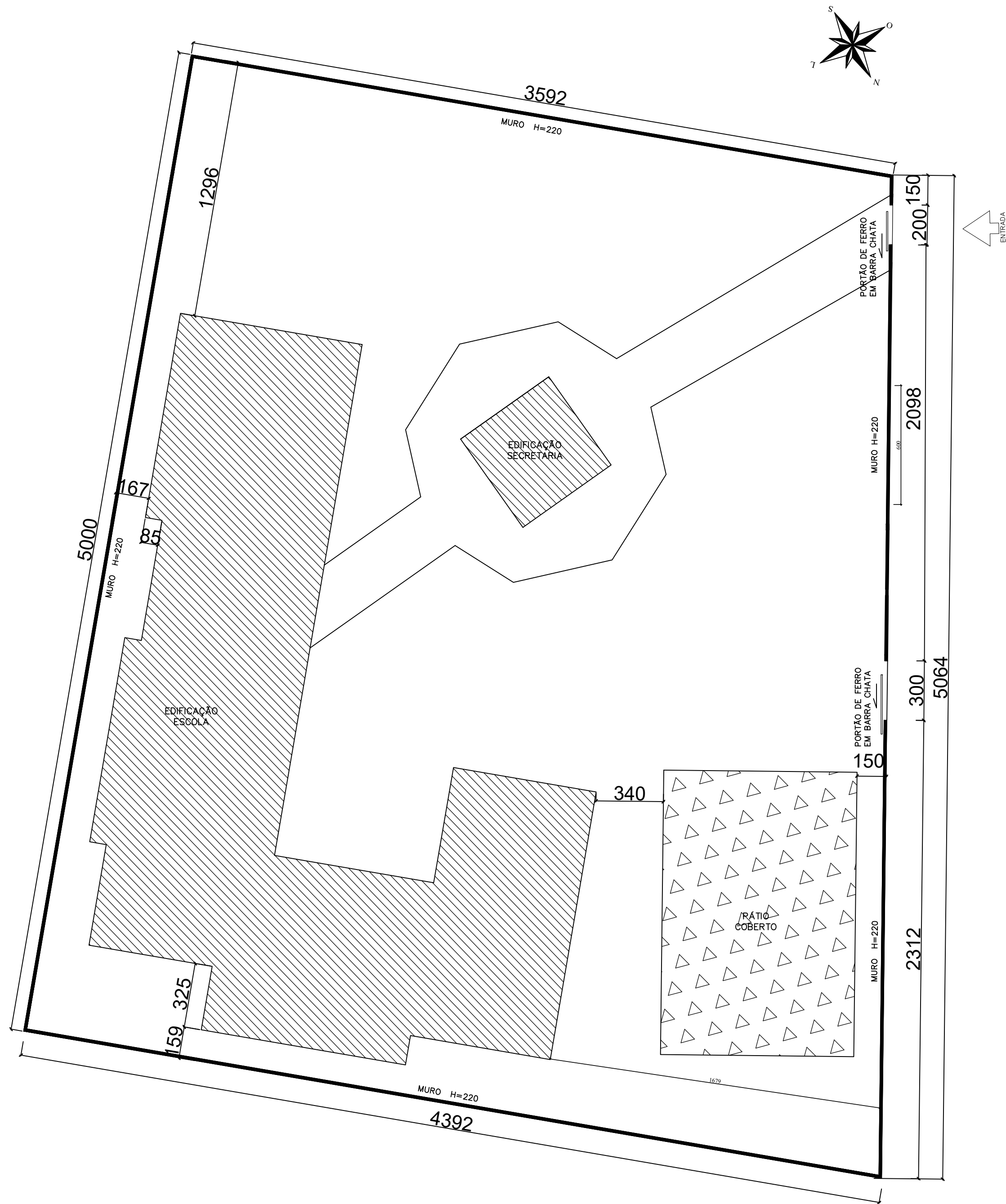
IMPLANTAÇÃO ESC.: 1/500
