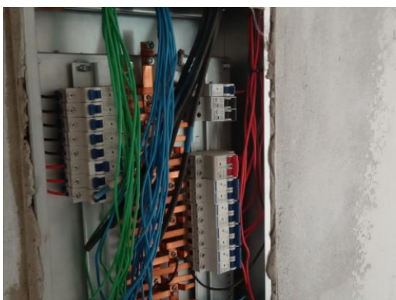
Foto 03 – Instalação dos disjuntores.
