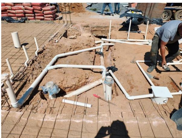
Foto 03 – Instalação de tubos e conexões enterradas.
