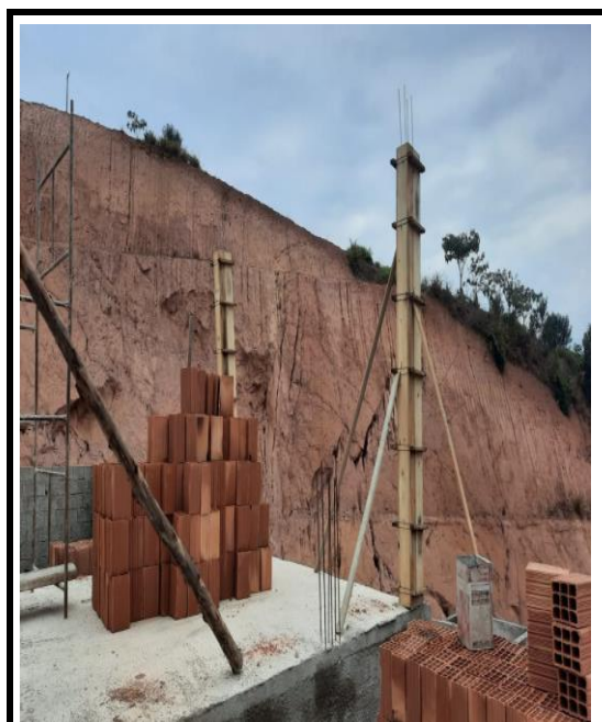
EXECUÇÃO DE ALVENARIA DA PLATIBANDA
