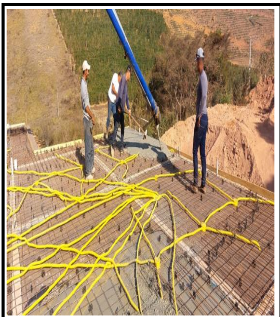
CONCRETAGEM DA LAJE
