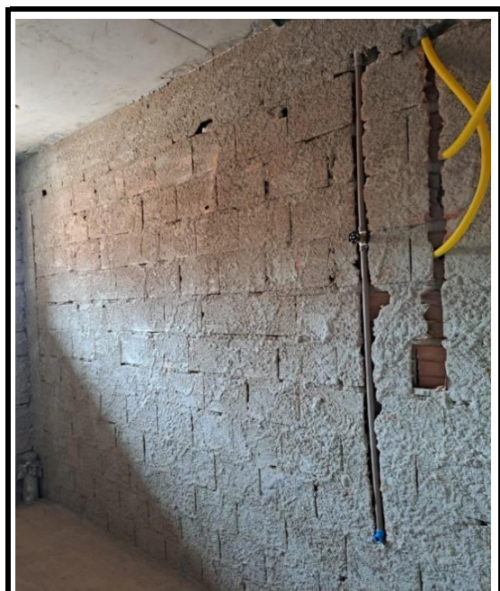
INSTALAÇÃO DE PONTOS DE ÁGUA FRIA
