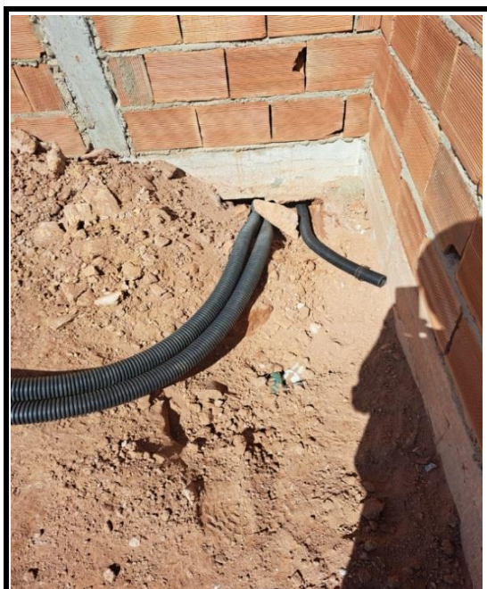
INSTALAÇÃO DE ELETRODUTO
