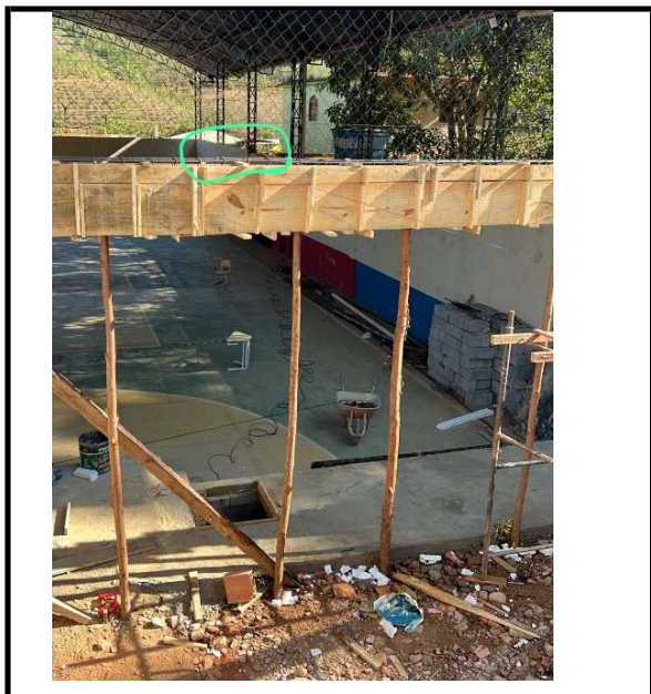
Figura 1 - Execução de Armação de Forma - Palco
