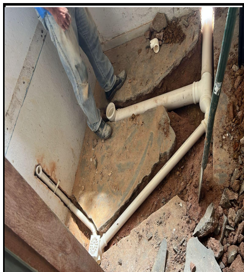
Figura 14 - tubo PVC de esgoto e Ralo
