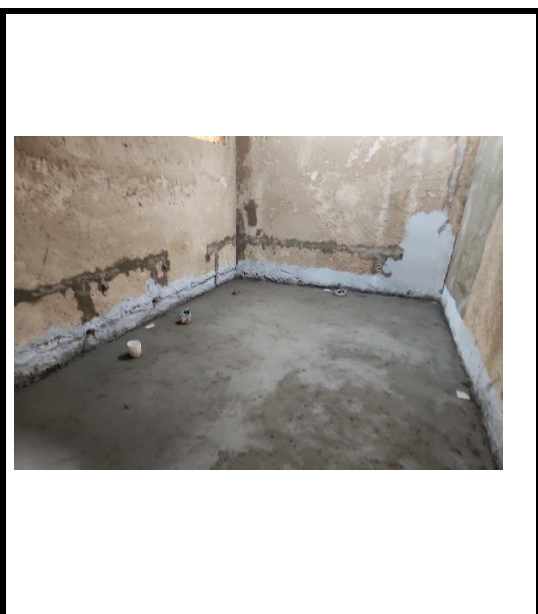
Impermeabilização polimérica
