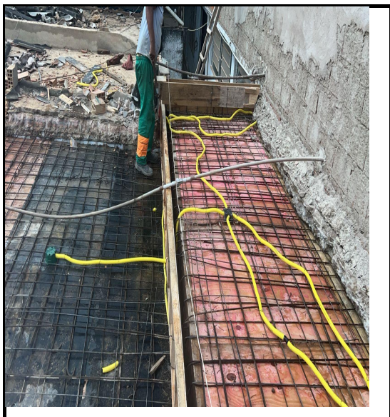
Figura 5 - Forma e Ferragem
