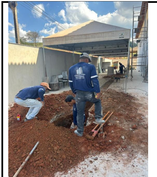
Figura 26- Abertura das cavas das caixas ralo de drenagem
