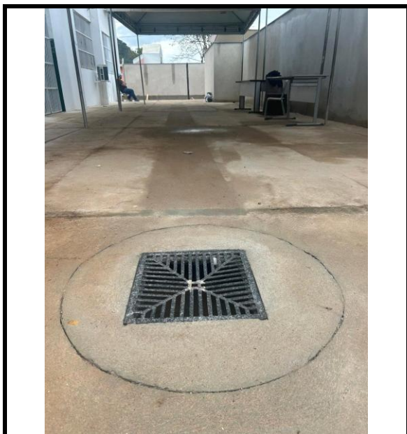
Figura 27 -chumbamento das caixas ralo de drenagem
