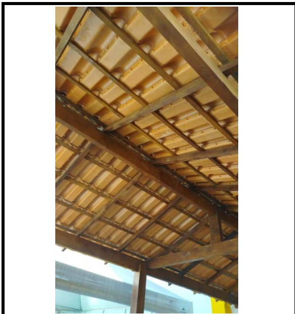
Figura 21 -Execução de madeiramento e de cobertura em telhas coloniais
