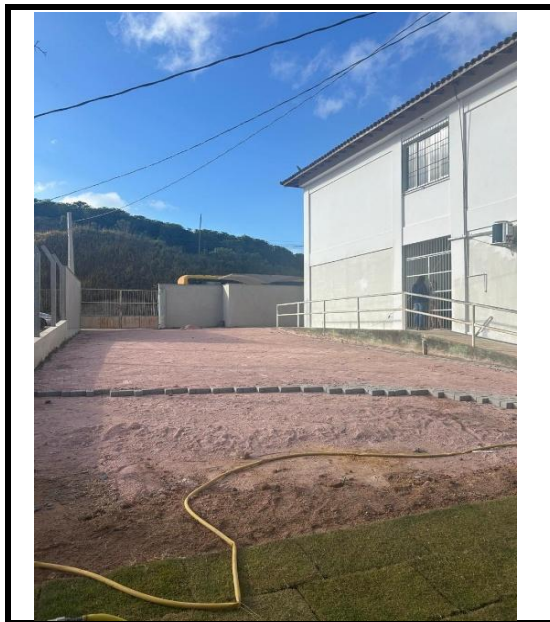
Figura 54- execução de calçamento com bloco holandes
