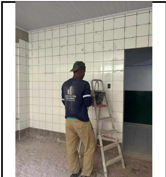
Figura 1 - Assentamento de pastilhas e rejuntamento
