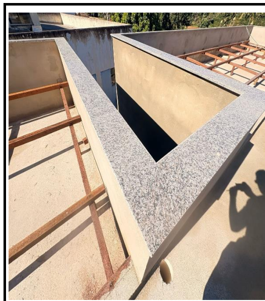
5.1.1 - Alvenaria de Blocos Cerâmicos / 5.3.1 - Verga/Contraverga Reta de Concreto
