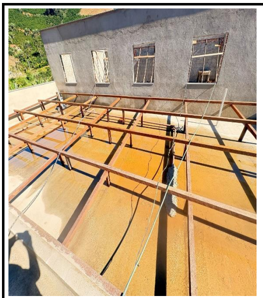
9.1.1 - Estrutura de Madeira de lei com pontaletes e caibros
