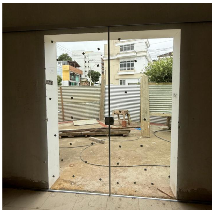
Foto 18 – Item 08.06 - Porta em vidro temperado 10mm, incolor, inclusive ferragens de fixação e instalação, exclusive puxador
