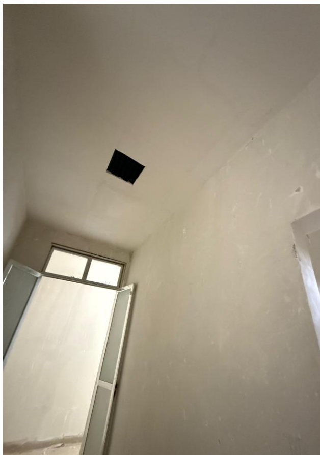
Fotos 24, 25 e 26 – Item 13.01 - Ponto padrão de luz no teto - considerando eletroduto PVC rígido de 3/4" inclusive conexões (4.5m), fio isolado PVC de 2.5mm 2 (16.2m) e caixa PVC 4x4" (1 und)
