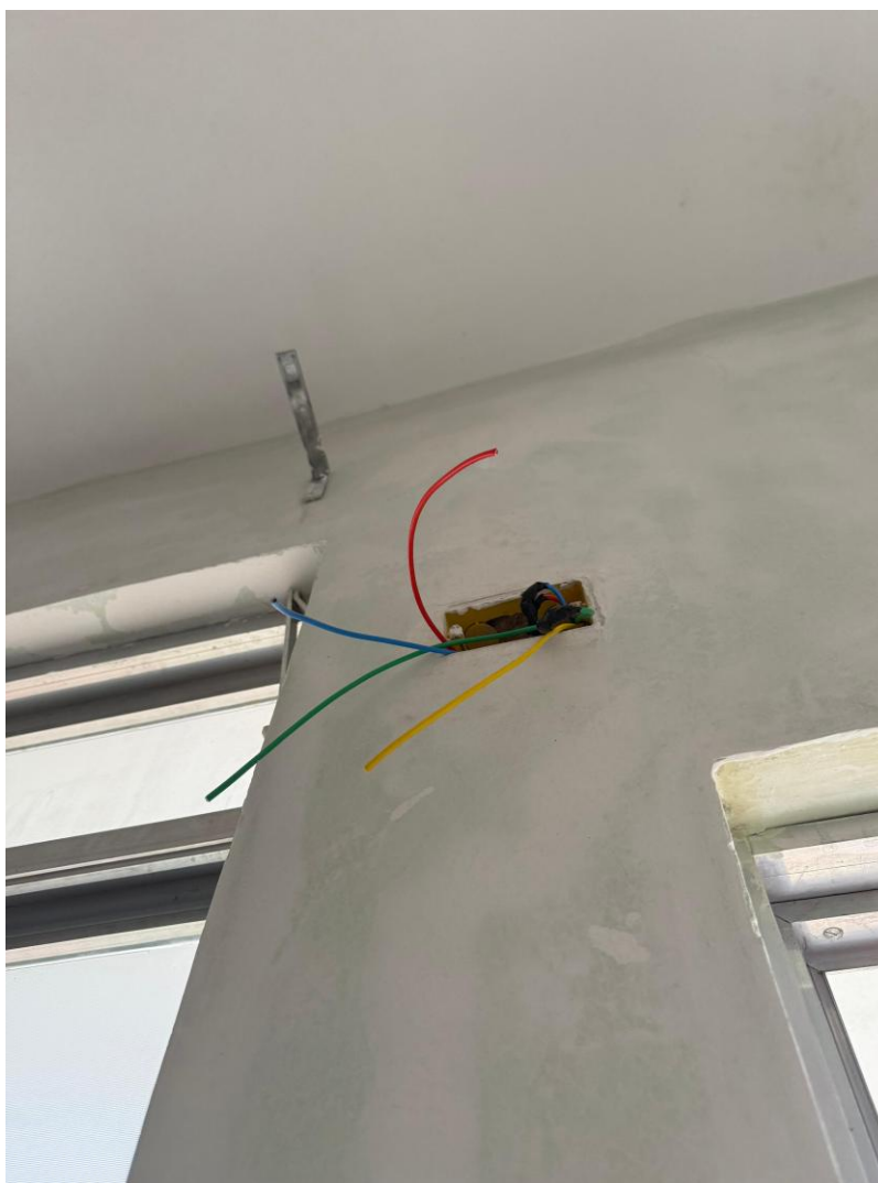
Fotos 29 e 30 – Item 13.04 - Ponto padrão de tomada para ar refrigerado - considerando eletroduto PVC rígido de 3/4" inclusive conexões (6.0m), fio isolado PVC de 4.0mm 2 (21.6m) e caixa PVC 4x2" (1 und)
