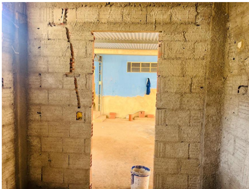
Fotos 03 e 04 – Item 05.01 - Verga/contraverga reta de concreto armado 10 x 5 cm, Fck = 15 MPa, inclusive forma, armação e desforma
