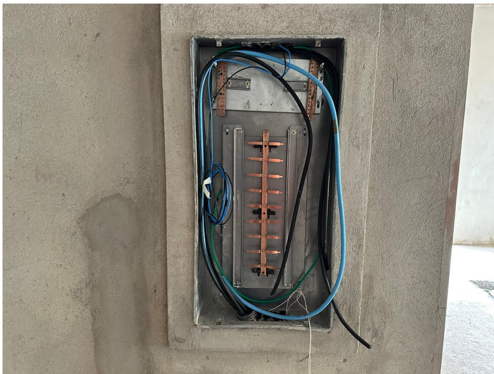
Instalação de quadro de distribuição e eletrodutos
