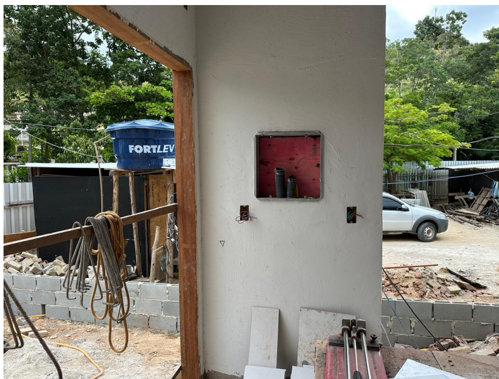
Instalação de quadro de distribuição para telefone eletrodutos
