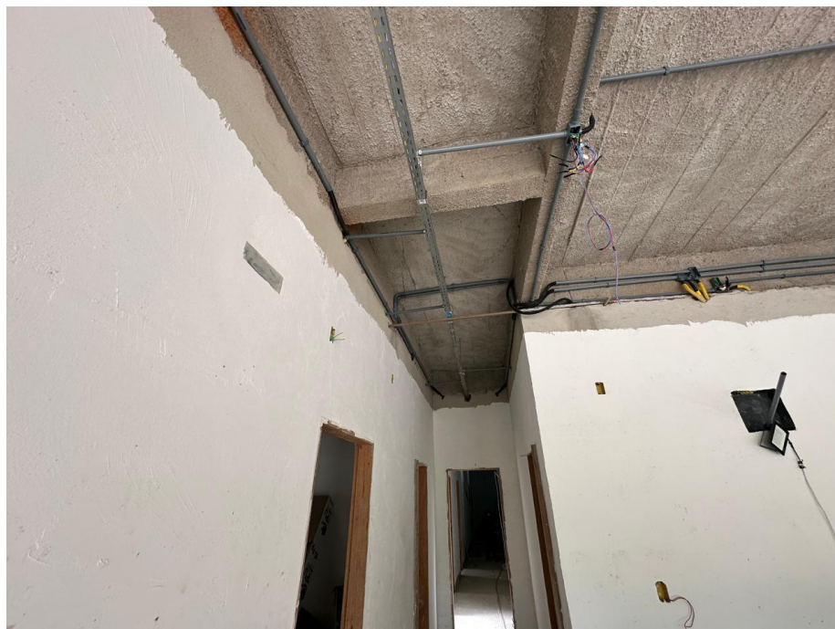
Instalação de infraestrutura de cabeamento estruturado e elétrica
