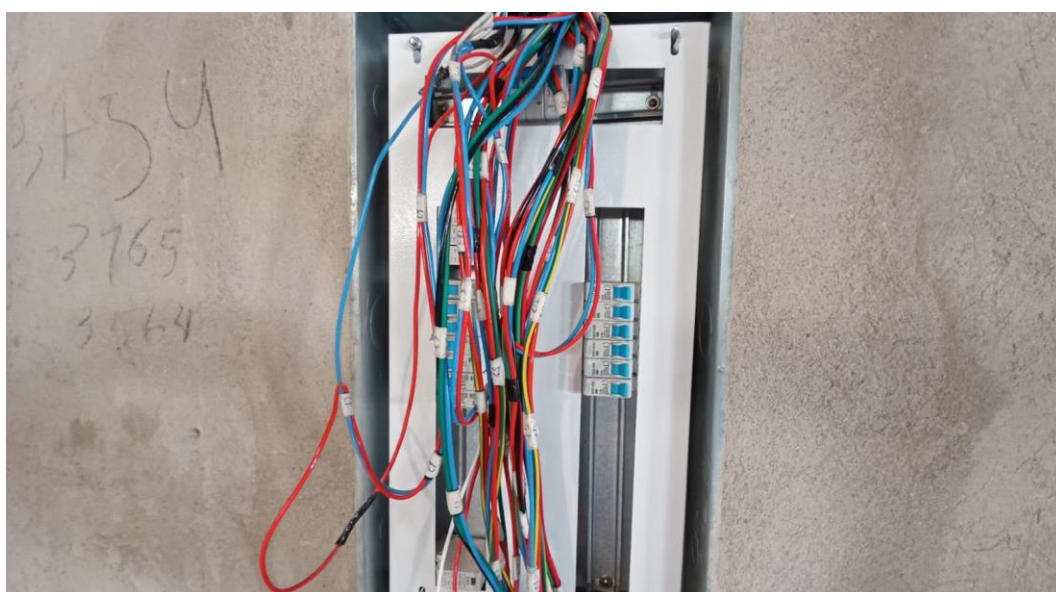
Figura 14 - Detalhe para cabos elétricos chegando até as caixas de distribuição – térreo e pavimento superior
