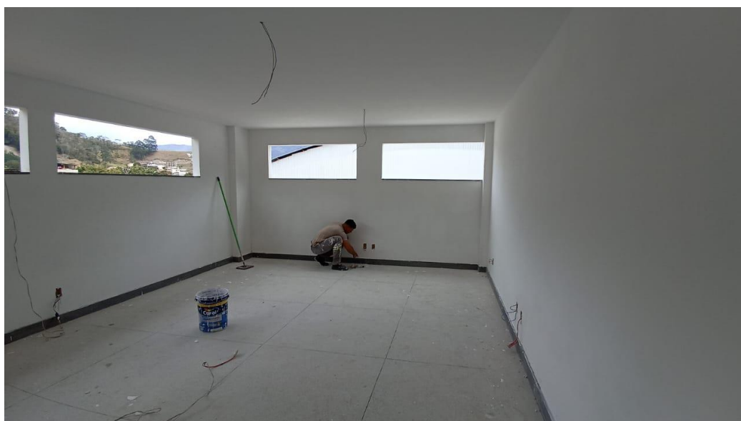
Figura 34 - Detalhe para emassamento das paredes – pavimento superior
