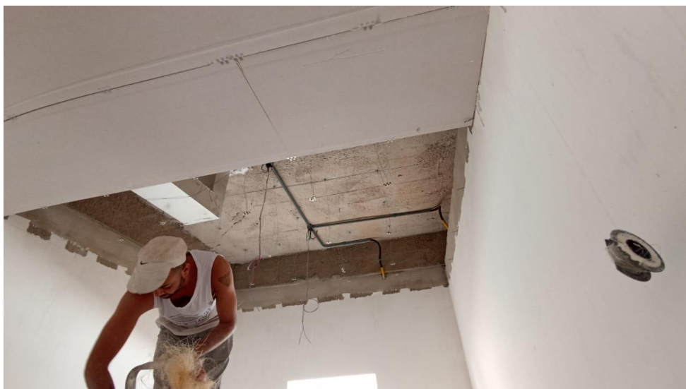
Figura 29 - Detalhe para execução do forro de gesso
