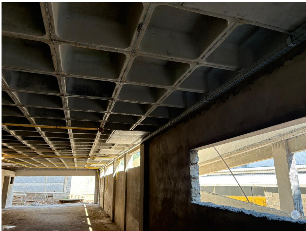
FOTO 05 – Eletrocalhas instaladas.
