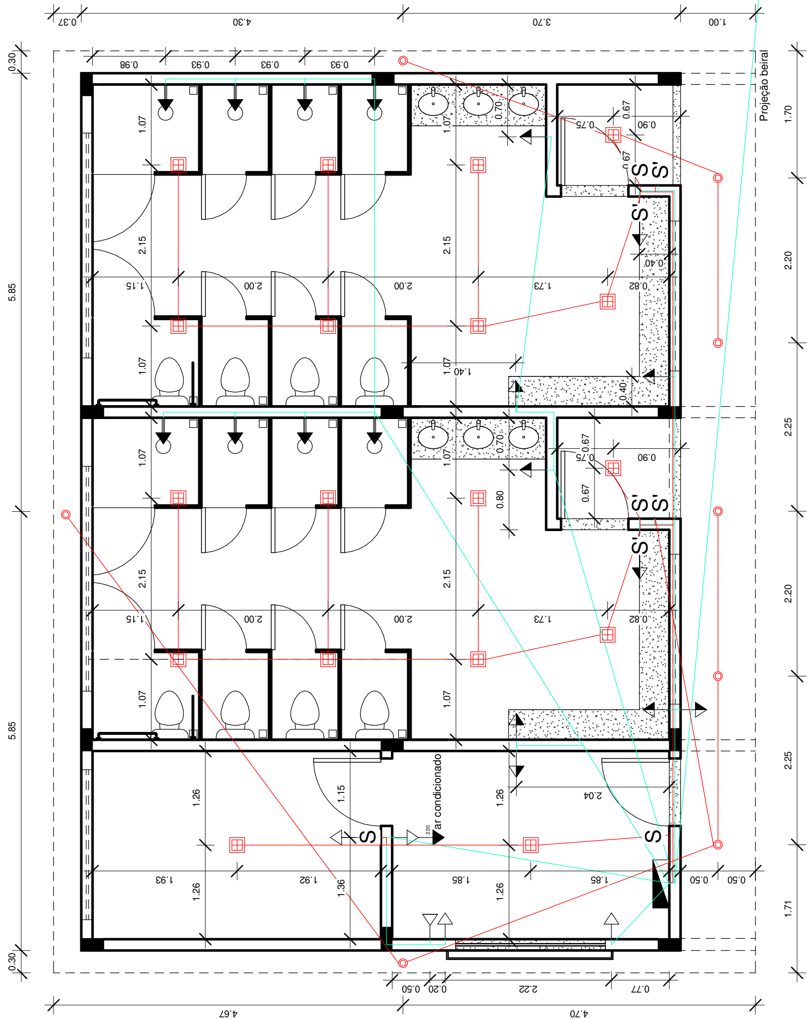
01 PROJETO ELÉTRICO 1 : 50
