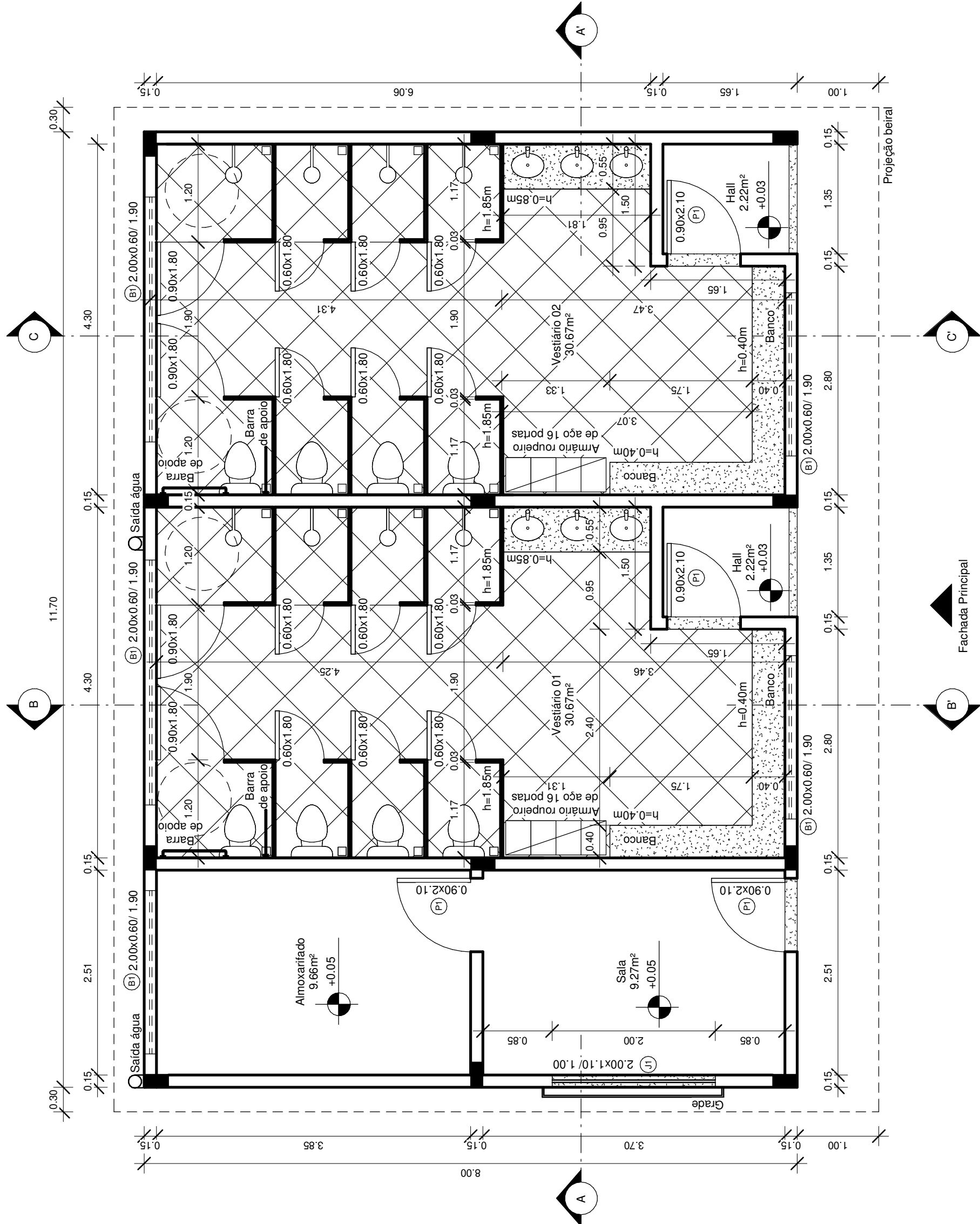
1 Planta Baixa
