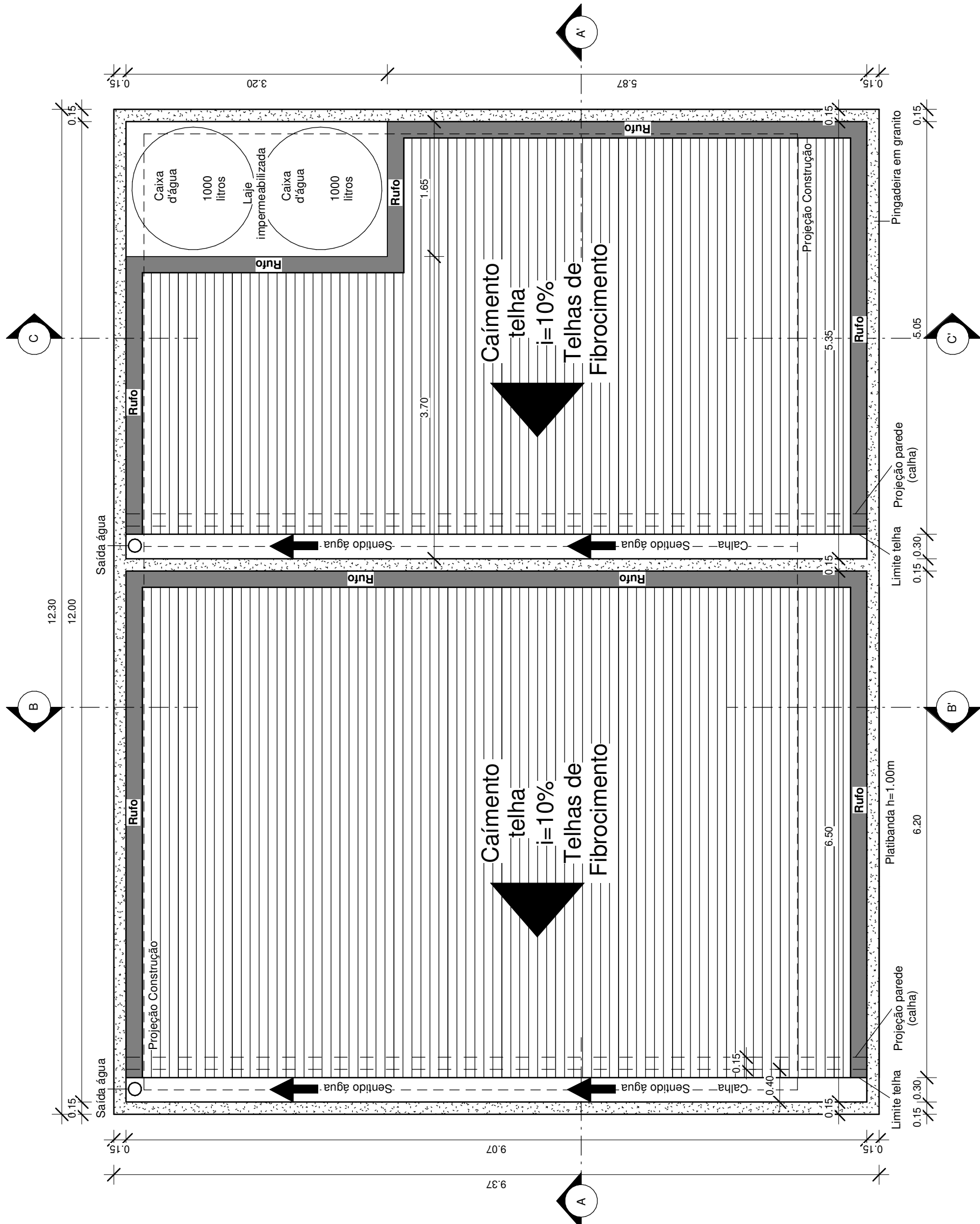
2 Planta de Cobertura
