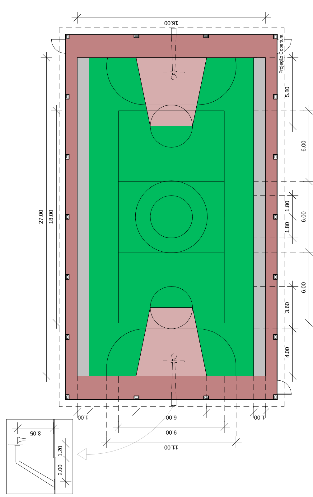
3 Detalhe quadra 1 : 200
