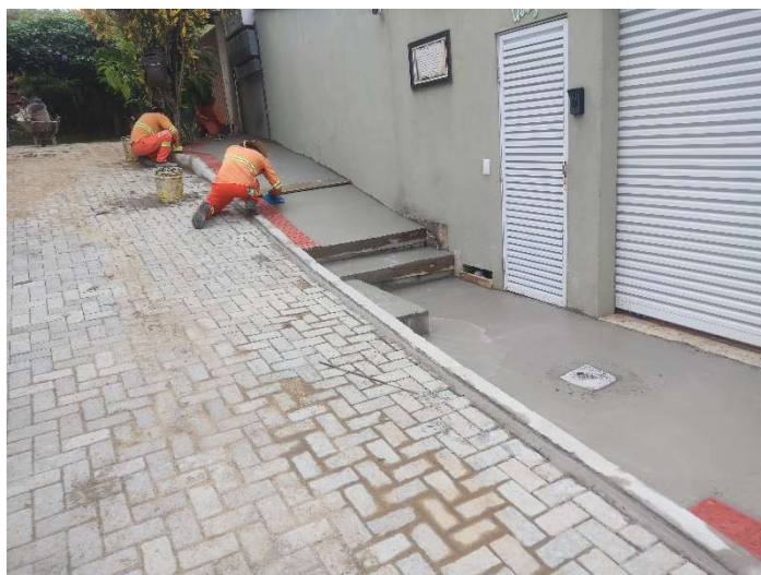
PASSEIO (CALÇADA) OU PISO DE CONCRETO COM CONCRETO MOLDADO IN LOCO, USINADO, ACABAMENTO CONVENCIONAL, ESPESSURA 6 CM, ARMADO
