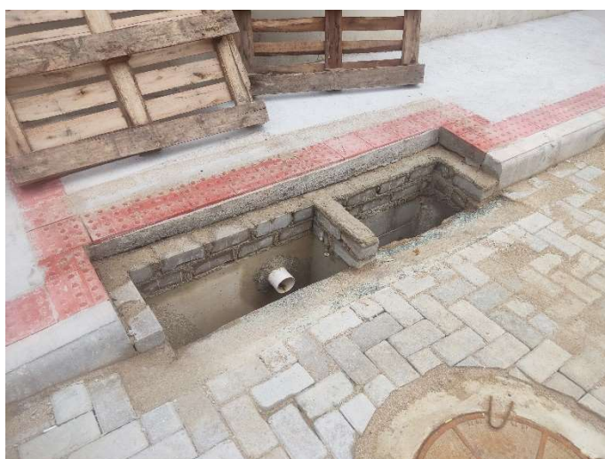
BOCA DE LOBO SIMPLES
