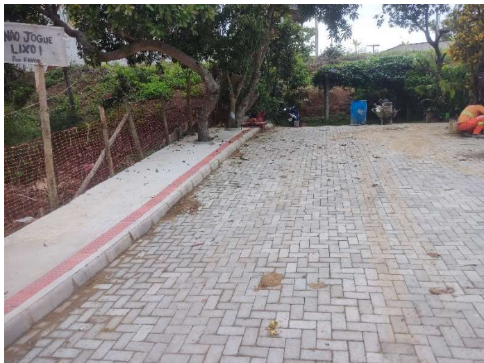
PAVIMENTAÇÃO COM BLOCOS DE CONCRETO (35 MPA), ESP.= 08 CM, COLCHÃO AREIA ESP.= 5CM
