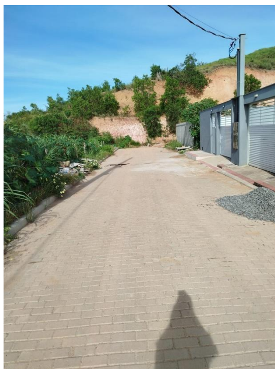
PAVIMENTAÇÃO COM BLOCOS DE CONCRETO (35 MPA), ESP.= 08 CM, COLCHÃO AREIA ESP.= 5CM
