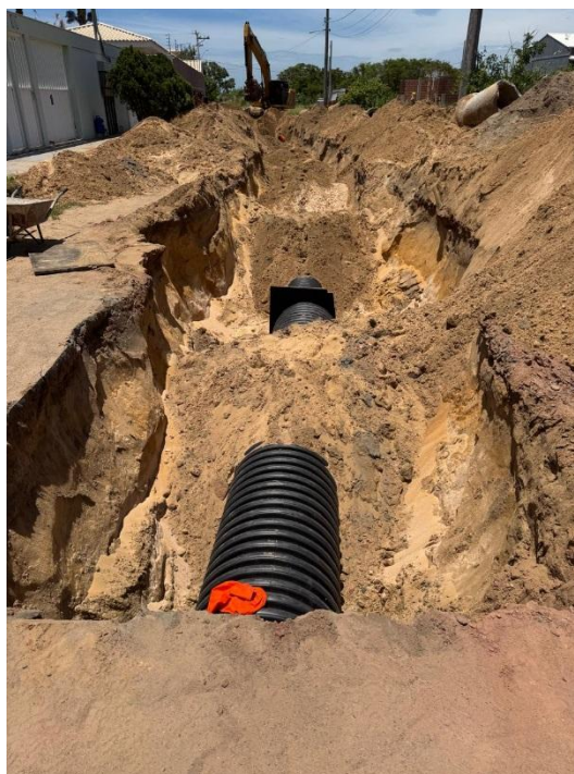
REATERRO COM AREIA
