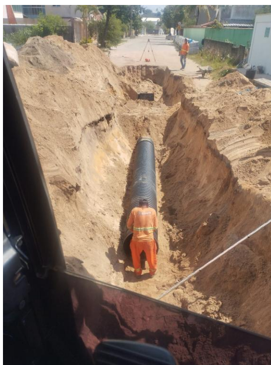
TUBO PEAD PARA DRENAGEM - D = 600 MM - FORNECIMENTO E INSTALAÇÃO
