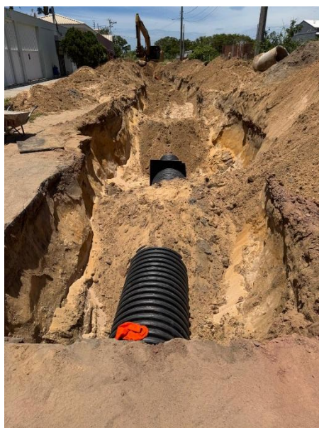
TUBO PEAD PARA DRENAGEM - D = 800 MM - FORNECIMENTO E INSTALAÇÃO
