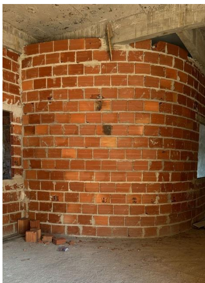
Figura 42: ALVENARIA DE BLOCOS CERÂMICOS 10 FUROS 10X20X20CM, ASSENTADOS C/ARGAMASSA DE CIMENTO, CAL HIDRATADA CH1 E AREIA TRAÇO 1:0,5:8, ESP. DAS JUNTAS 12MM E ESP. DAS PAREDES S/REVESTIMENTO, 10CM (BLOCO COMPRADO NA FÁBRICA, POSTO OBRA)
