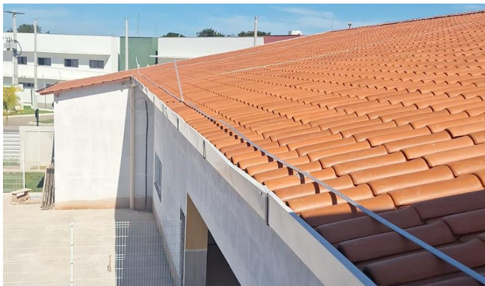
Figura 26: BARRA CHATA EM ALUMÍNIO 7/8"X1/8" (70MM 2 ), COM FUROS DIÂMETRO 7 MM REF. TEL-771, MARCA DE REFERÊNCIA TERMOTÉCNICA OU EQUIVALENTE
