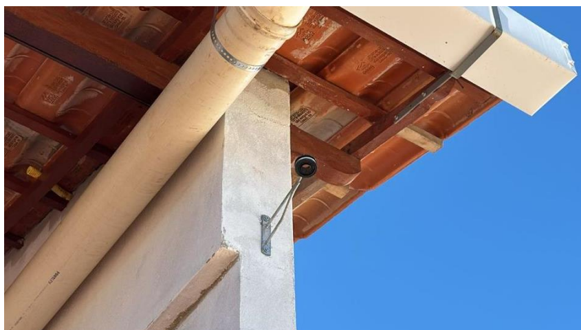
Figura 29: TERMINAL ESTANHADO DE 1 COMPRESSÃO 1 FURO, 50MM², REF. TEL-5150, MARCA DE REFERÊNCIA TERMOTÉCNICA OU EQUIVALENTE
