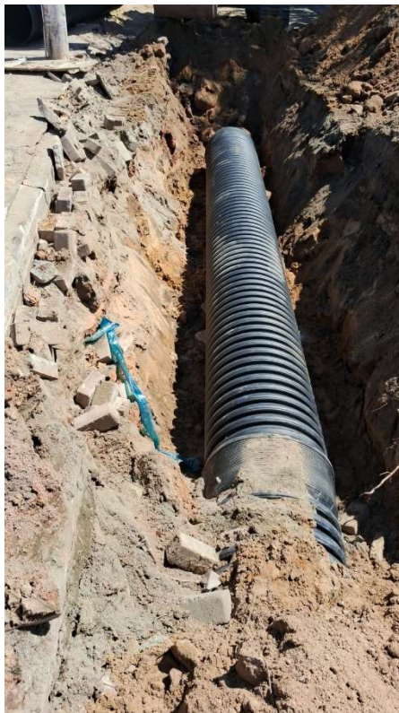
TUBO PEAD PARA DRENAGEM - D = 600 MM - FORNECIMENTO E INSTALAÇÃO
