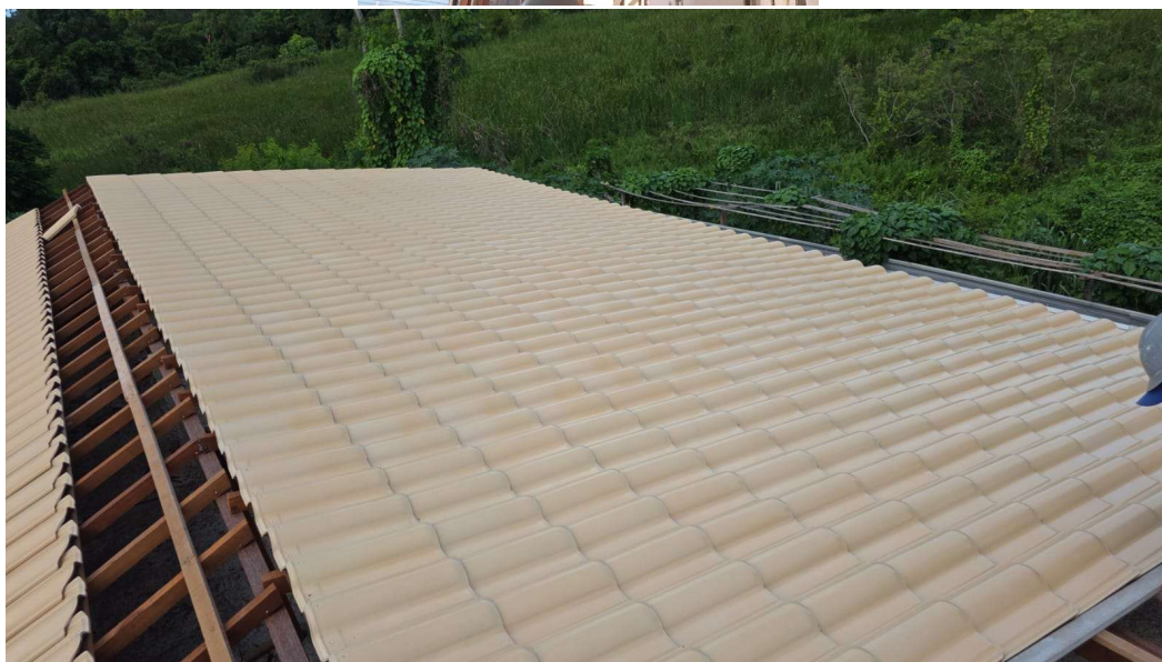
COBERTURA NOVA DE TELHAS CERÂMICAS TIPO CAPA E CANAL INCLUSIVE CUMEEIRAS (TELHAS COMPRADAS NA FÁBRICA, POSTO OBRA)
