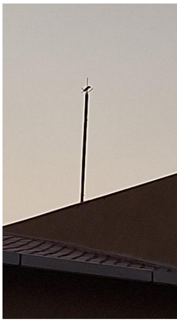
Figura 1: PÁRA-RAIOS TIPO FRANKLIM INCLUINDO BASE DE FIXAÇÃO, CONJUNTO DE CONTRAVENTAGEM C/ABRAÇADEIRA P/3 ESTAIS EM TUBO E DEMAIS ACESSÓRIOS C/EXCEÇÃO DO CABO DE COBRE DE DESCIDA E SUPORTES ISOLADORES
