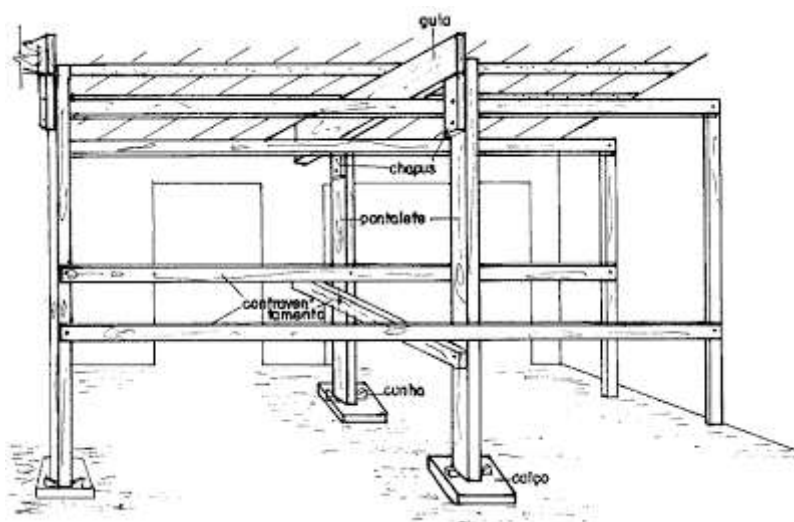
Figura 1- Exemplo de escoramento para laje pré-fabricada
