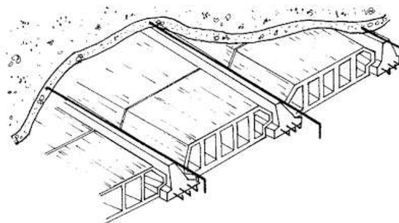
Figura 3 - Detalhe da colocação da armadura negativa
