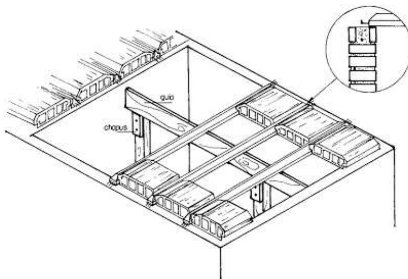
Figura 2 - Detalhe da colocação da laje pré-fabricada
