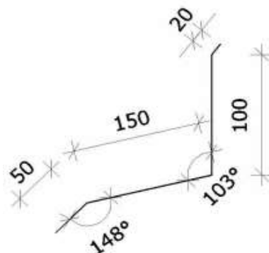
Figura 5 - Detalhamento do rufo
