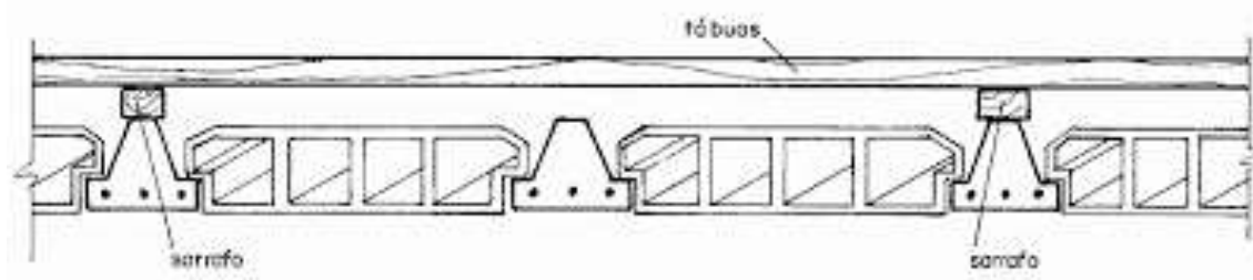
Figura 4 - Tábuas para passeio
