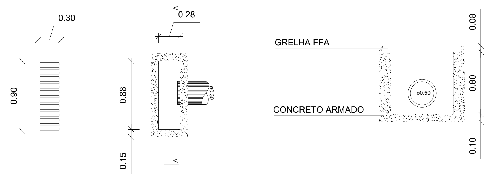
DET. CAIXA RALO ( D.I 0.28 x 0.88 x 0.80) ESC. 1/50
