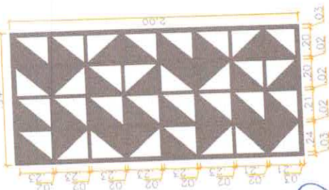
Vista Frontal Grade 01 em metal pintado com chapas em alumínio preto fosco
