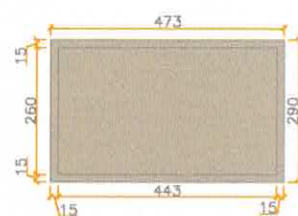
Vista Posterior
