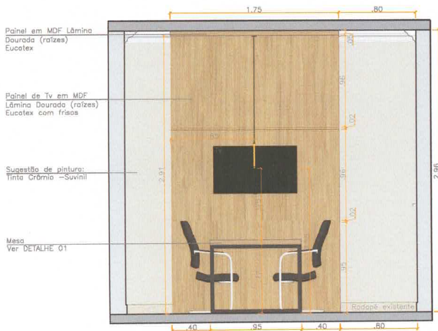
Vista 02 Escala 1/25
