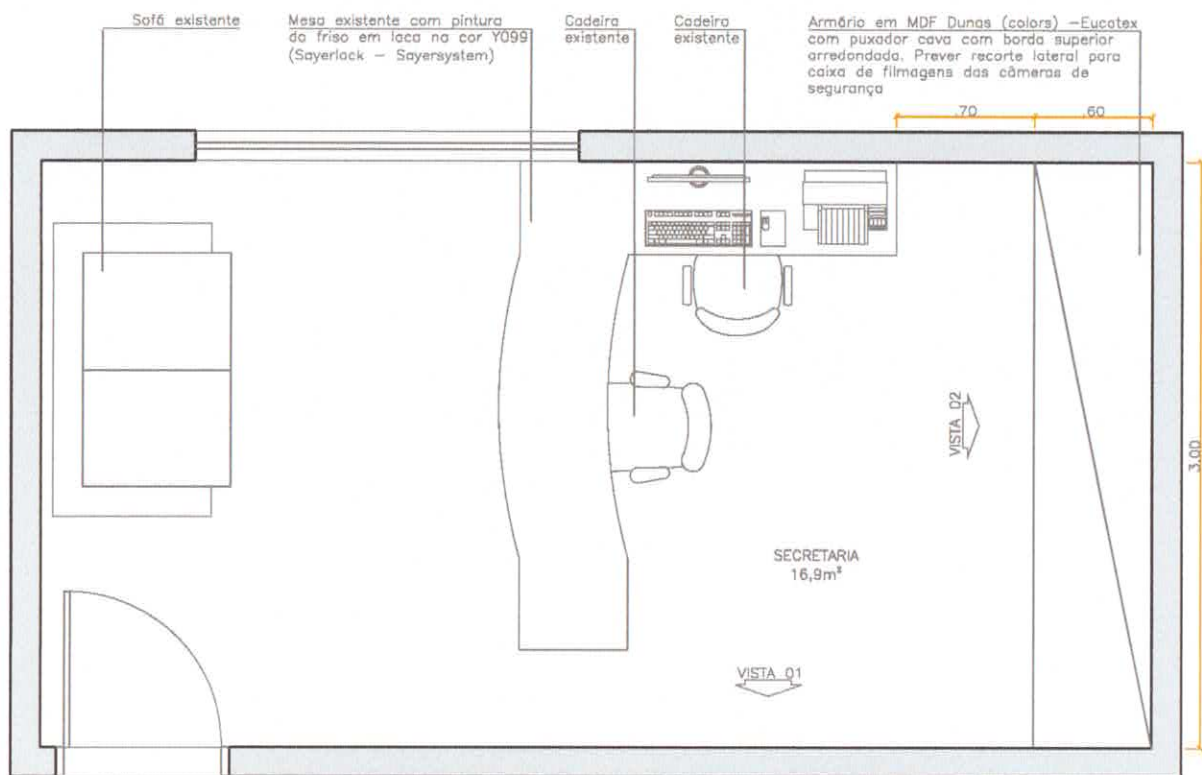
Planta de Layout Escala 1/25
