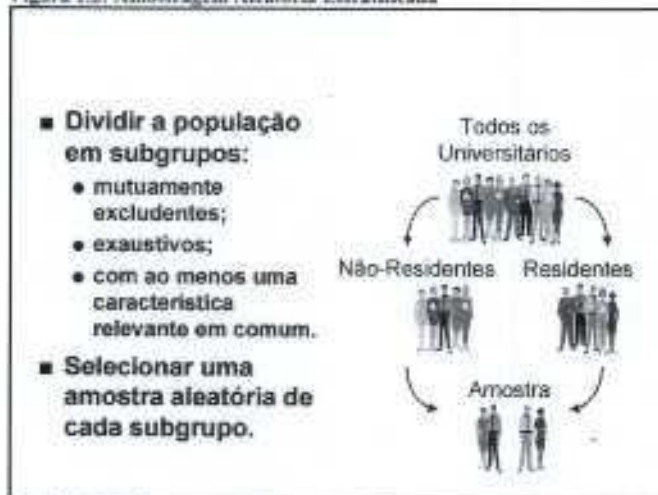
Figura 1.2: Amostragem Aleatória Estratificada
