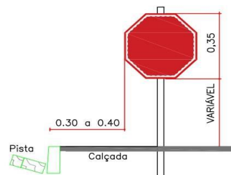
VISTA - OPÇÃO 01
