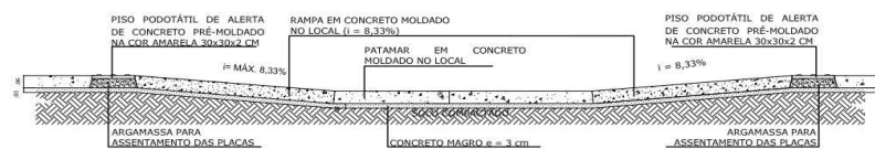
3 SEÇÃO A S/ ESCALA
