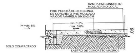
4 SEÇÃO B S/ ESCALA
