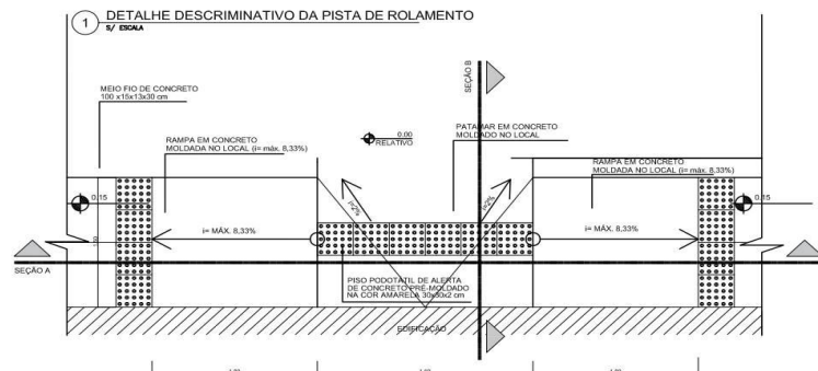
2 PLANTA BAIXA RAMPADA ACESSIBILIDADE S/ ESCALA
