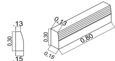
5 DETALHE MEIO FIO S/ ESCALA
